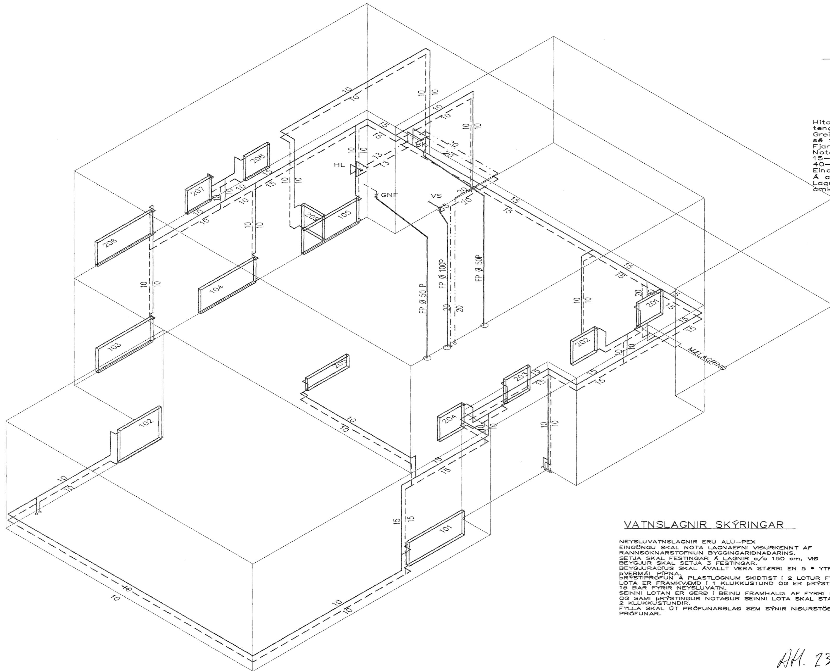
RÚMMYND HITA-VATNS OG FRÆRENNISLAGNA 1:50
