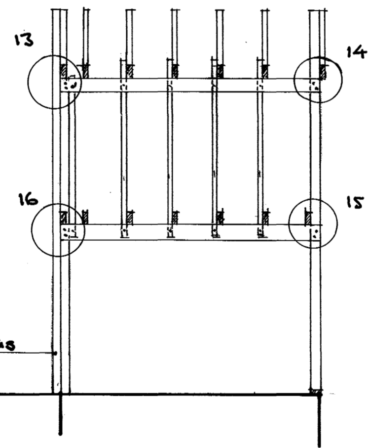
SNID B-B M 1:50
