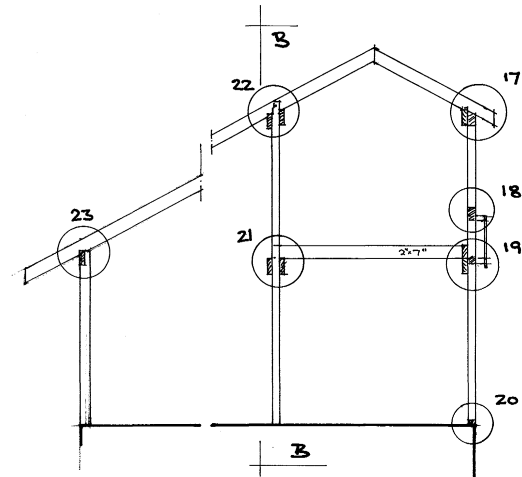
SNID A-A M 1:50
