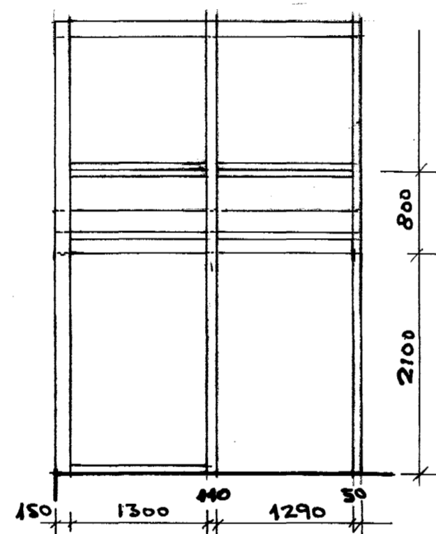
AUSTURHLID M 1:50
