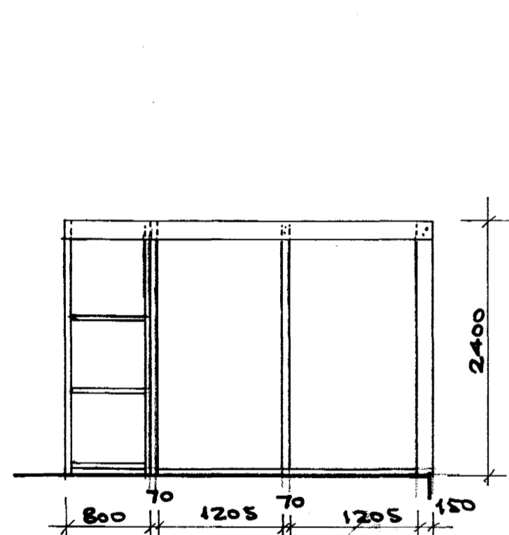
VESTURHLID M 1:50
