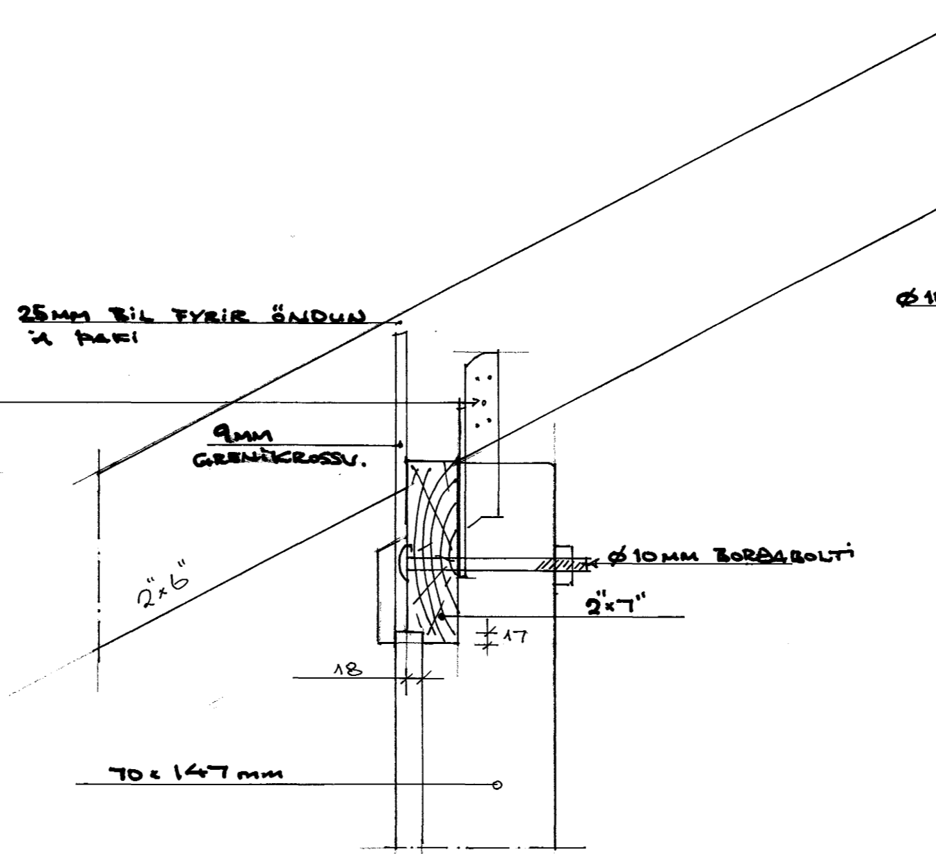
SÉRMYND NR 23 M 1:5
