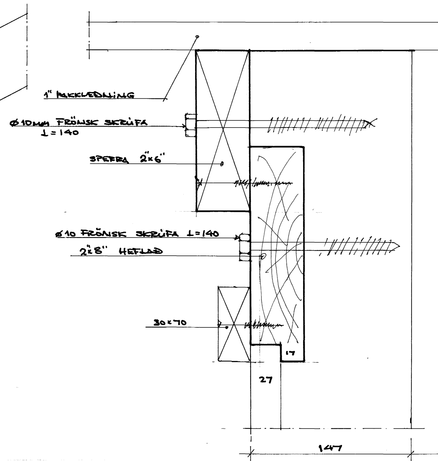
SNID C-C M 1:2
