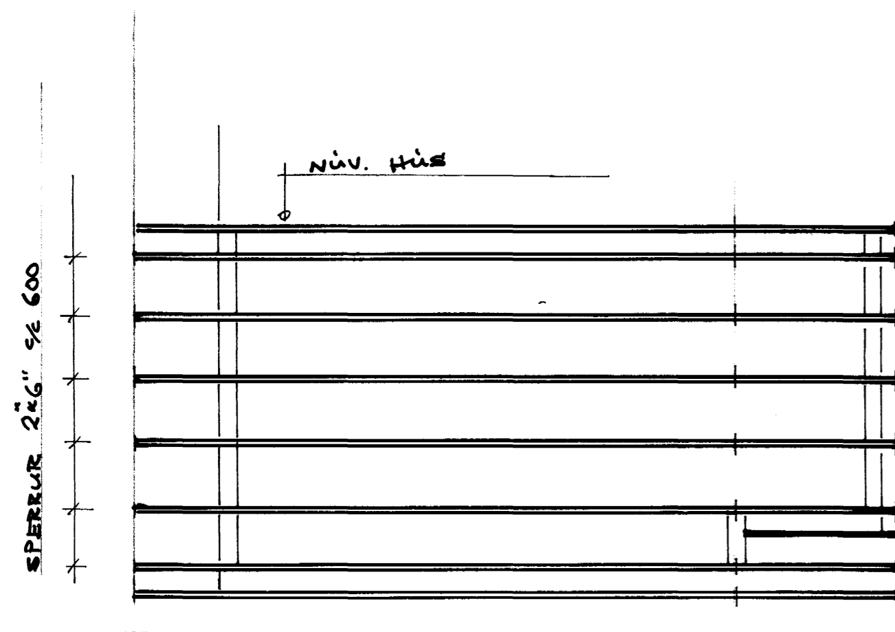
ÞAKVIÐIR M 1:50
