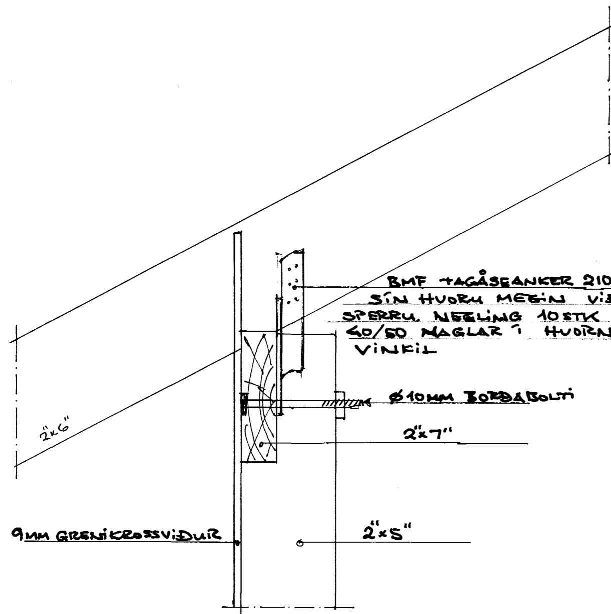
SÉRMYND NR 23 M 1:5
