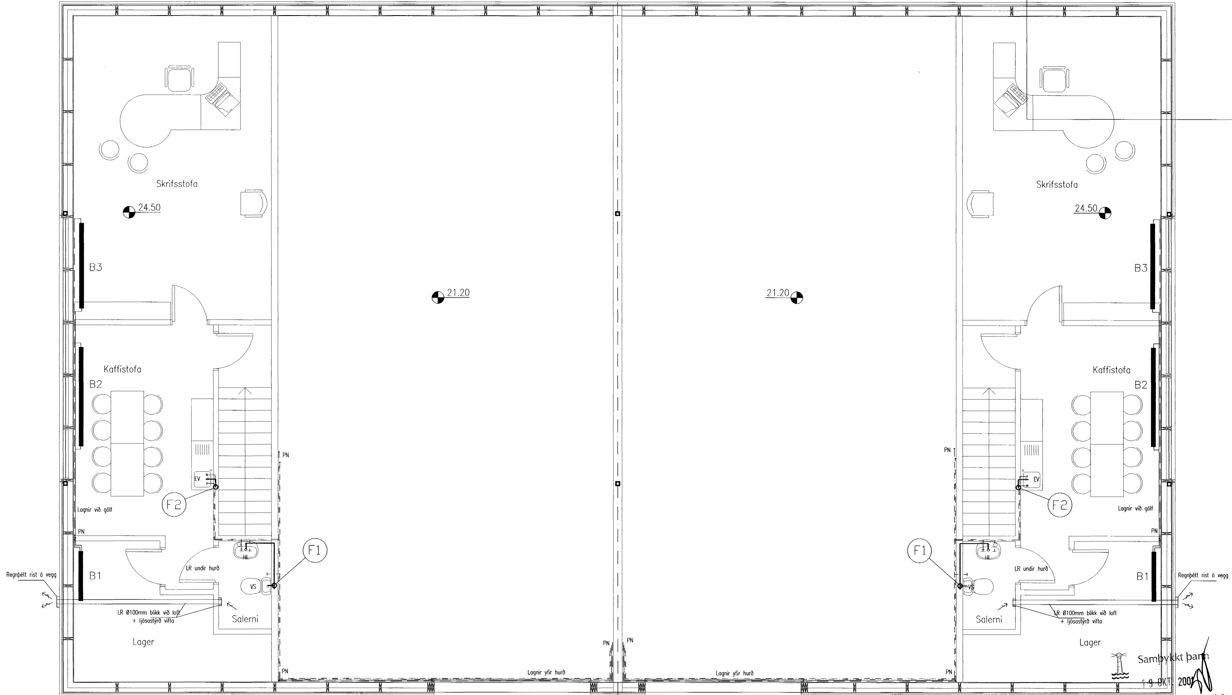
Grunnmynd millilofts 1:50
