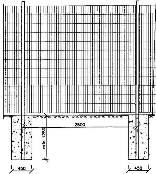
Snið 1 girðingu Mælikvarði 1: 20
