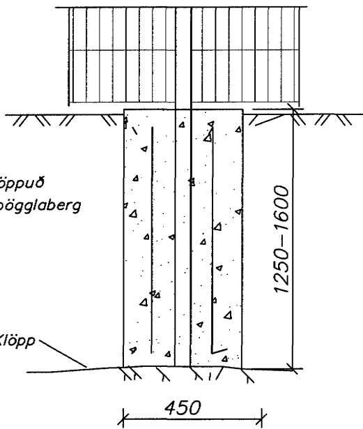
Snið 1 girðingu Mælikvarði 1: 20
