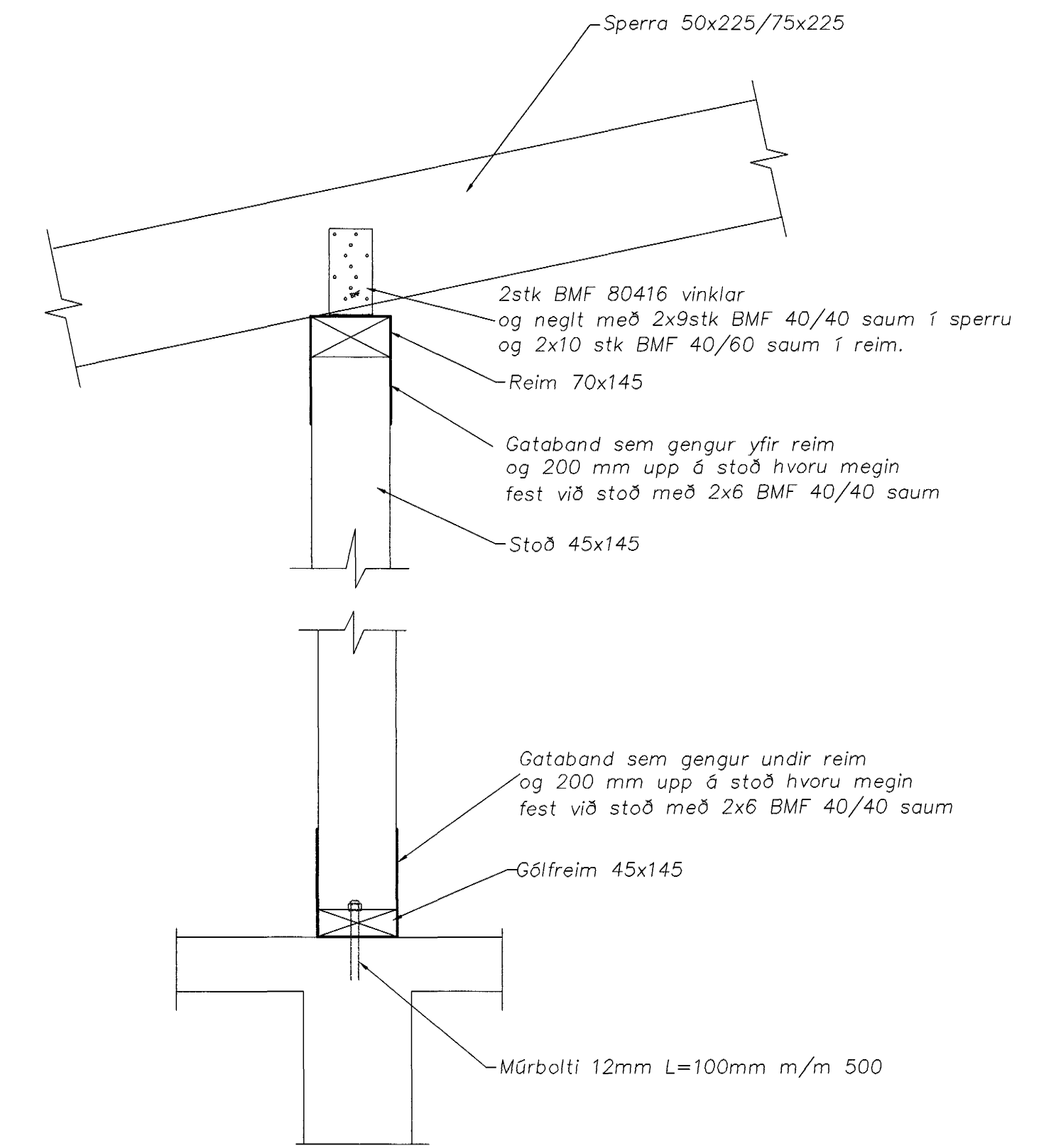
A bakvirki sérteikningar 209 Málkvörðir 1:10
