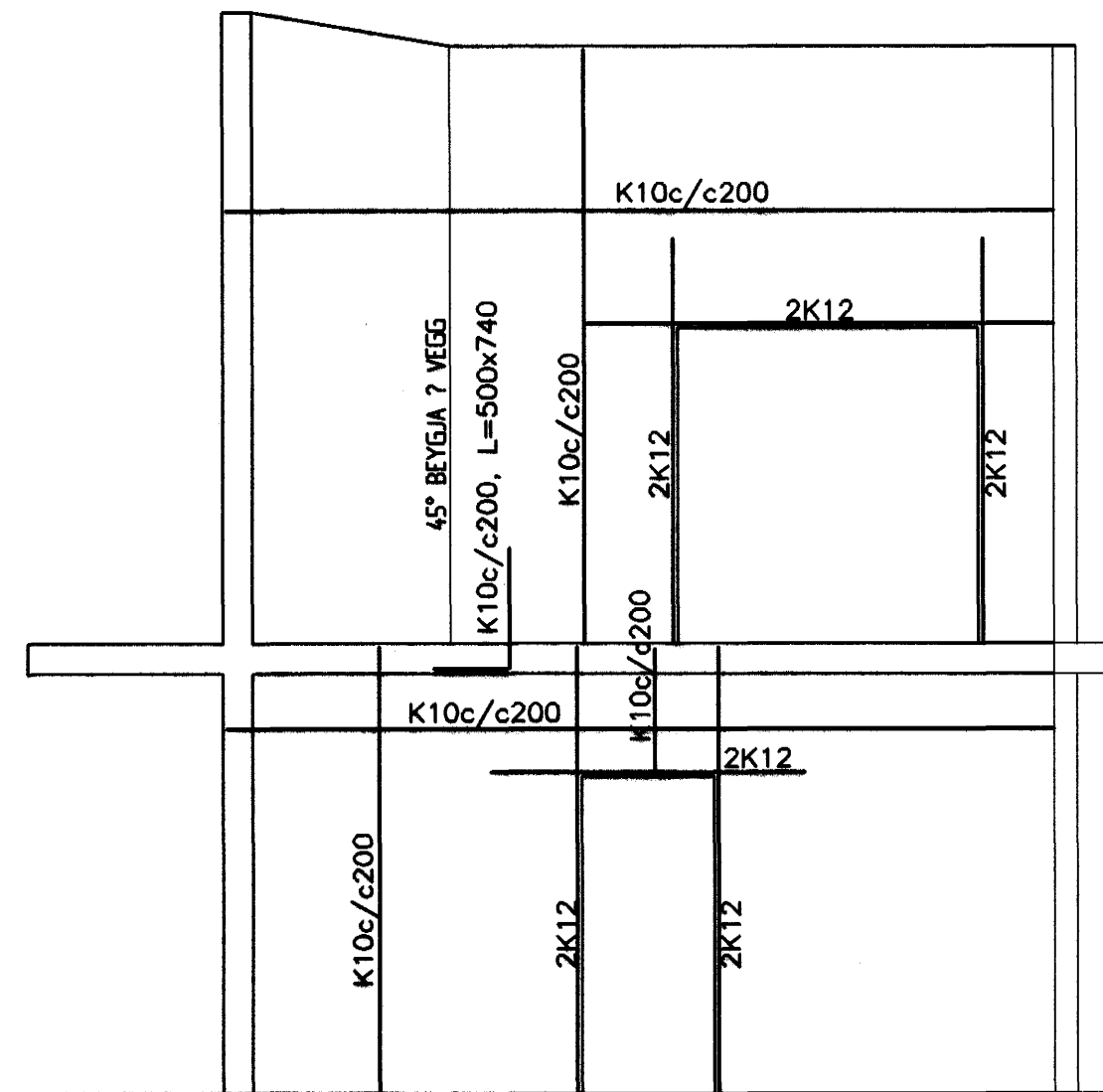
INNVEGGUR C 1:50
