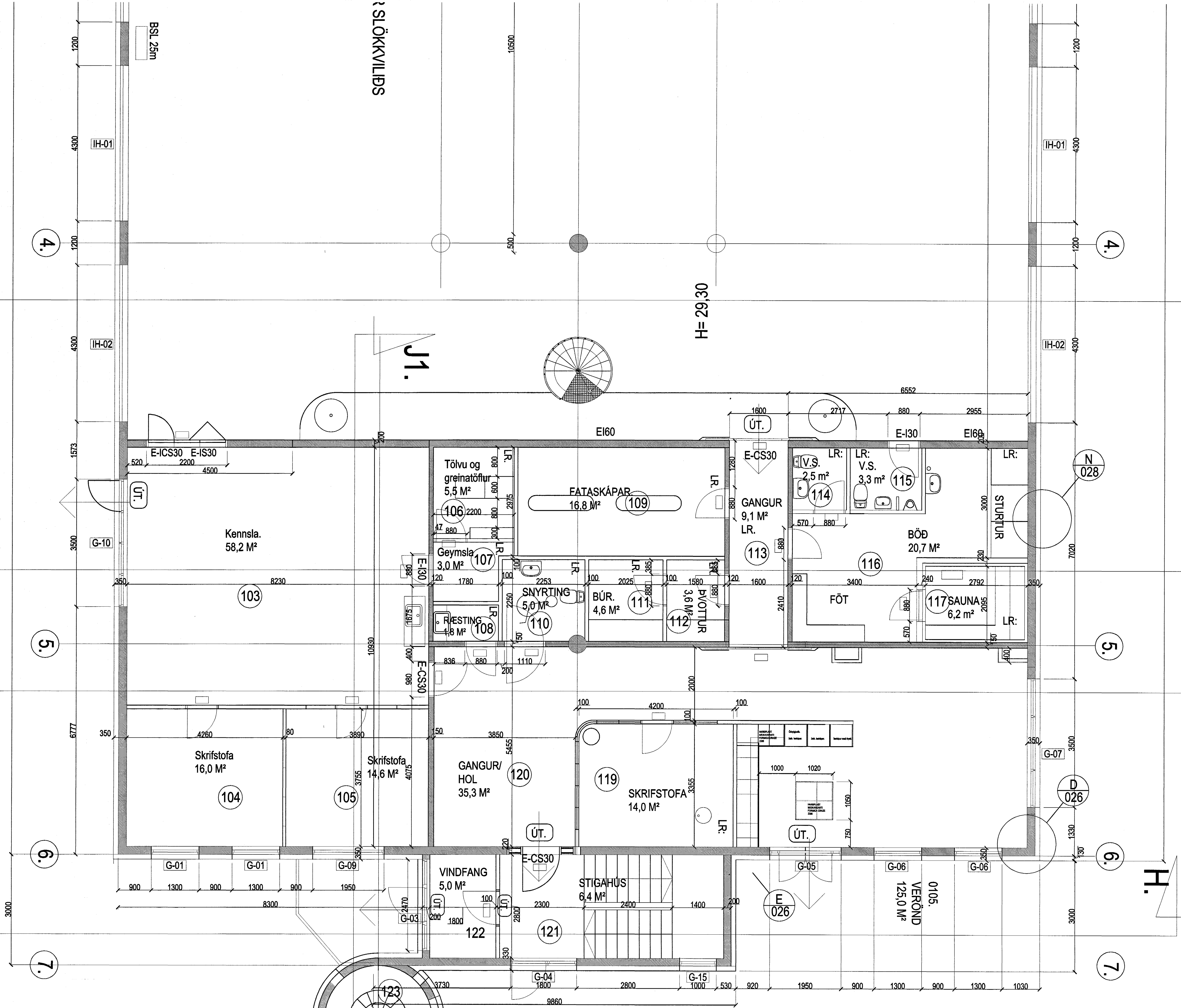
Grunnmynd 1. hæð. Mkv. 1:50 (Modull 3-7)
