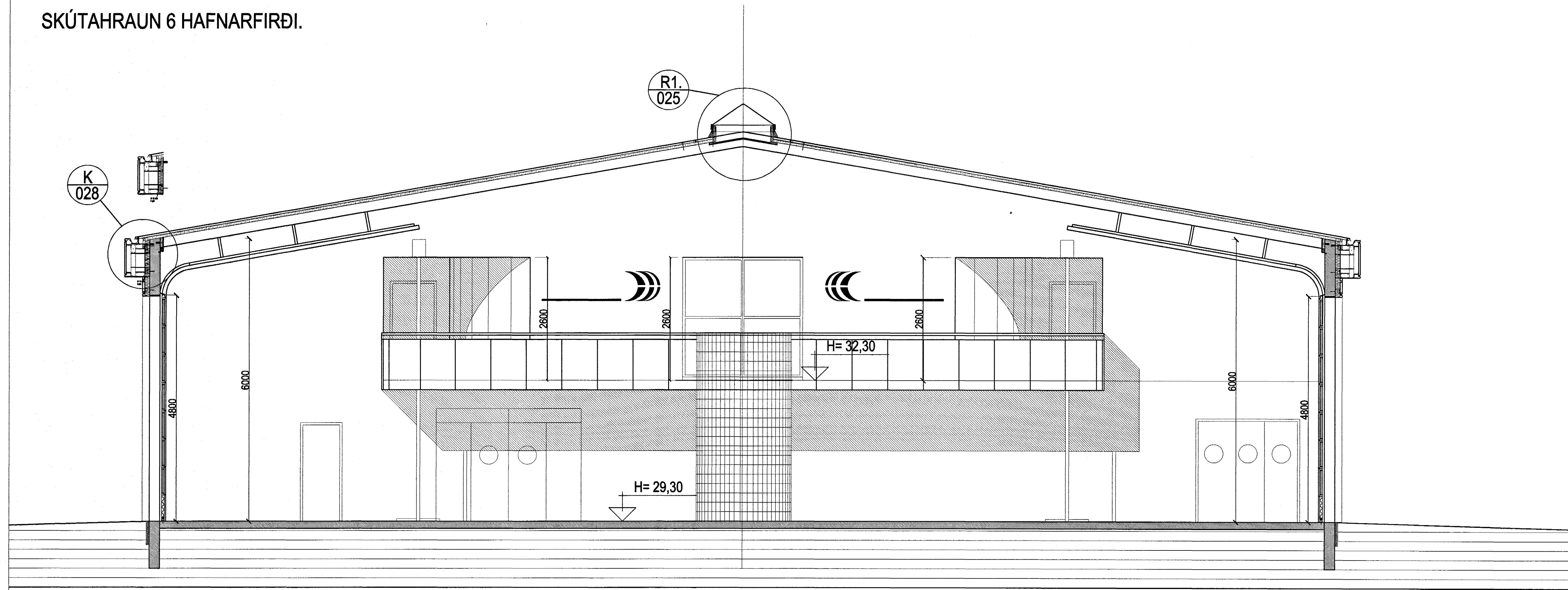
Snið A-A Mkv. 1:50.
