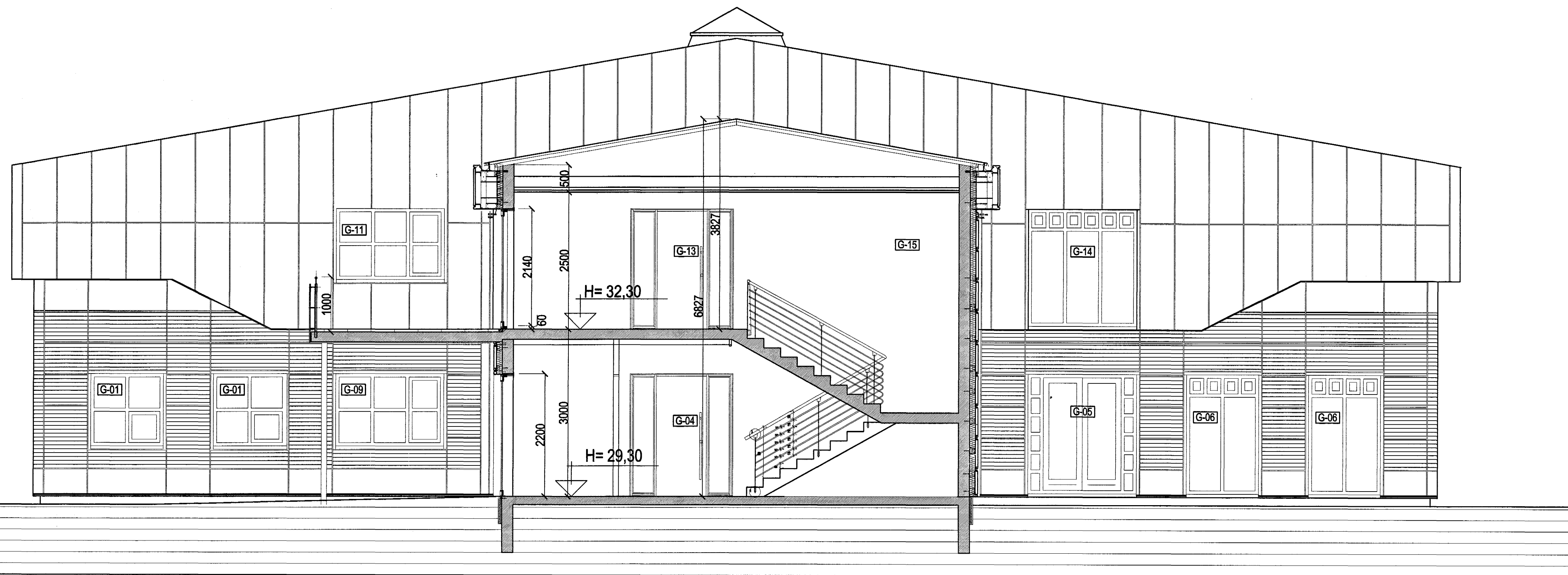
Snið H-H. Mkv. 1:50.
