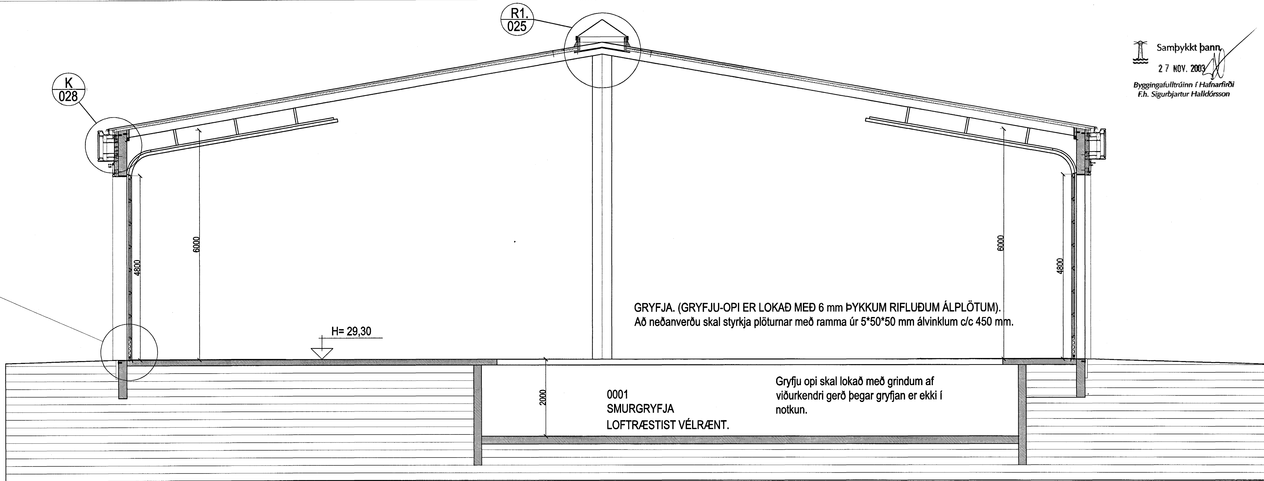
Snið I-I Mkv. 1:50.
