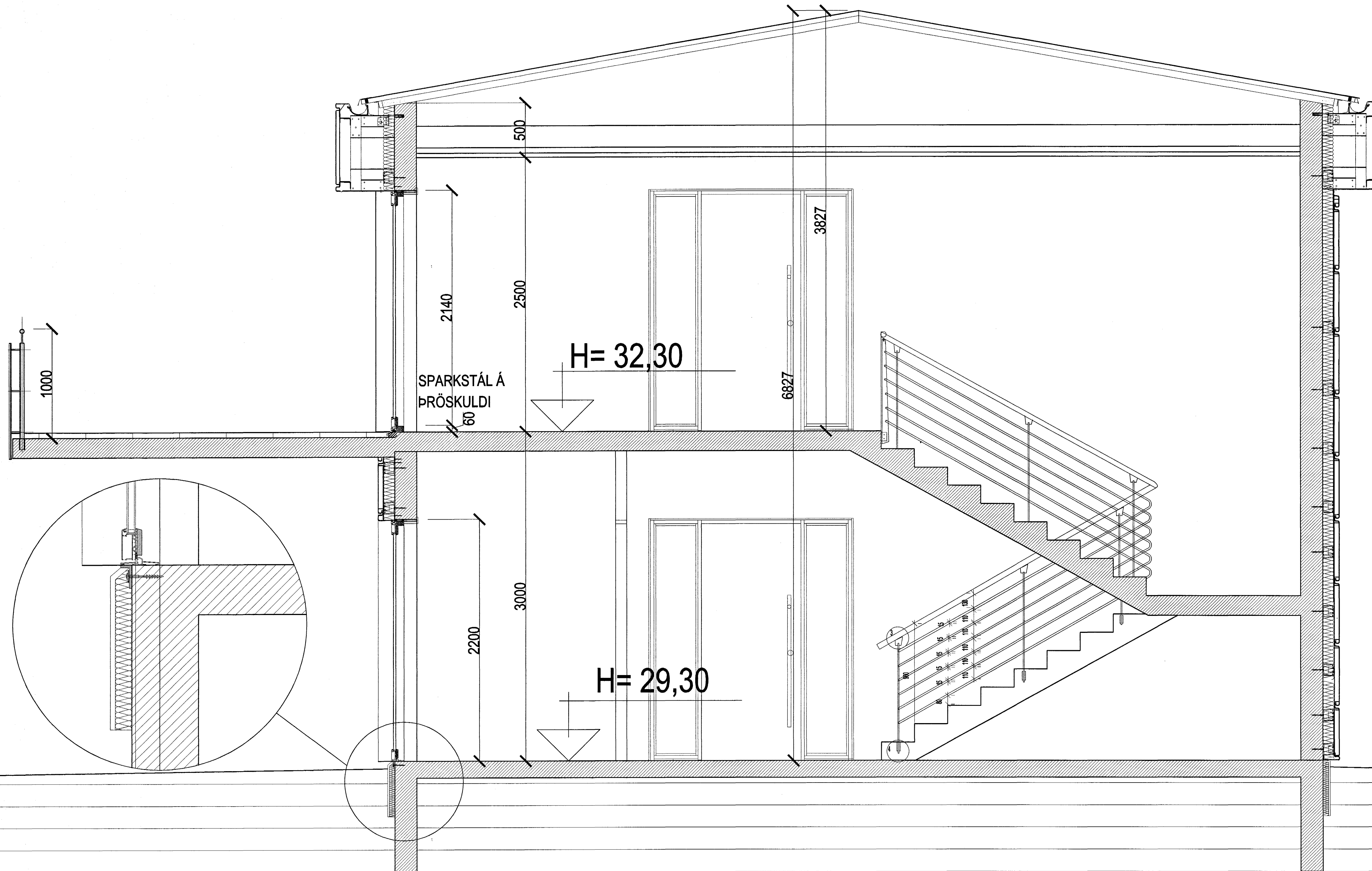
SNIÐ Í STIGAHÚS. MKV. 1:20.
