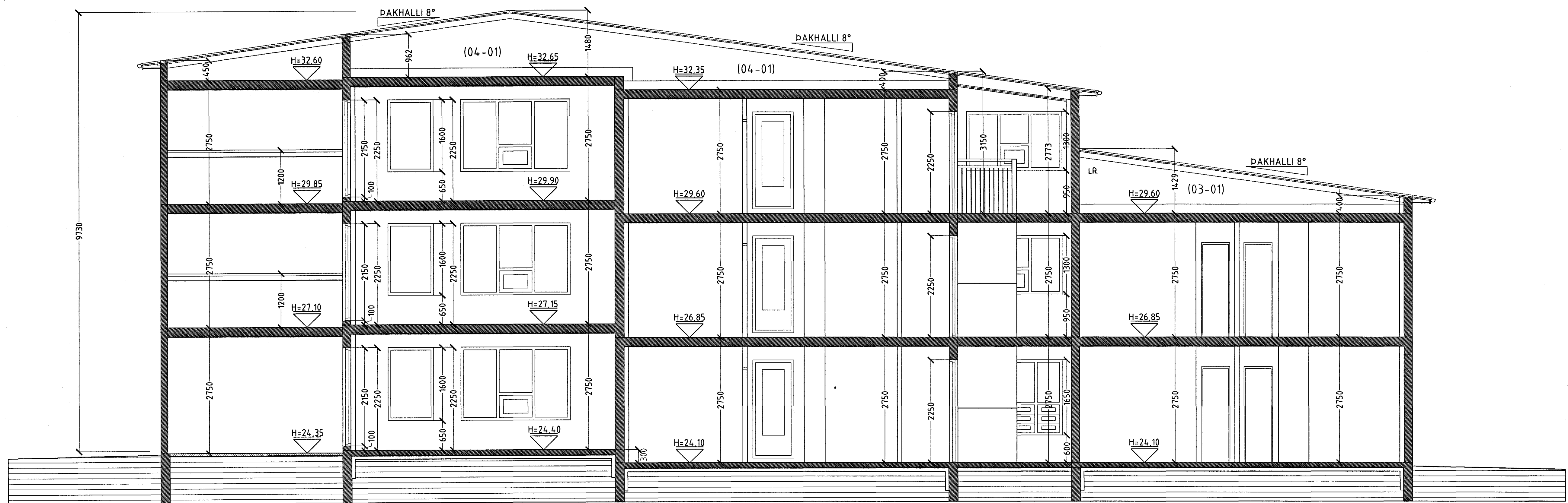
SNID C-C MKV. 1:50.
