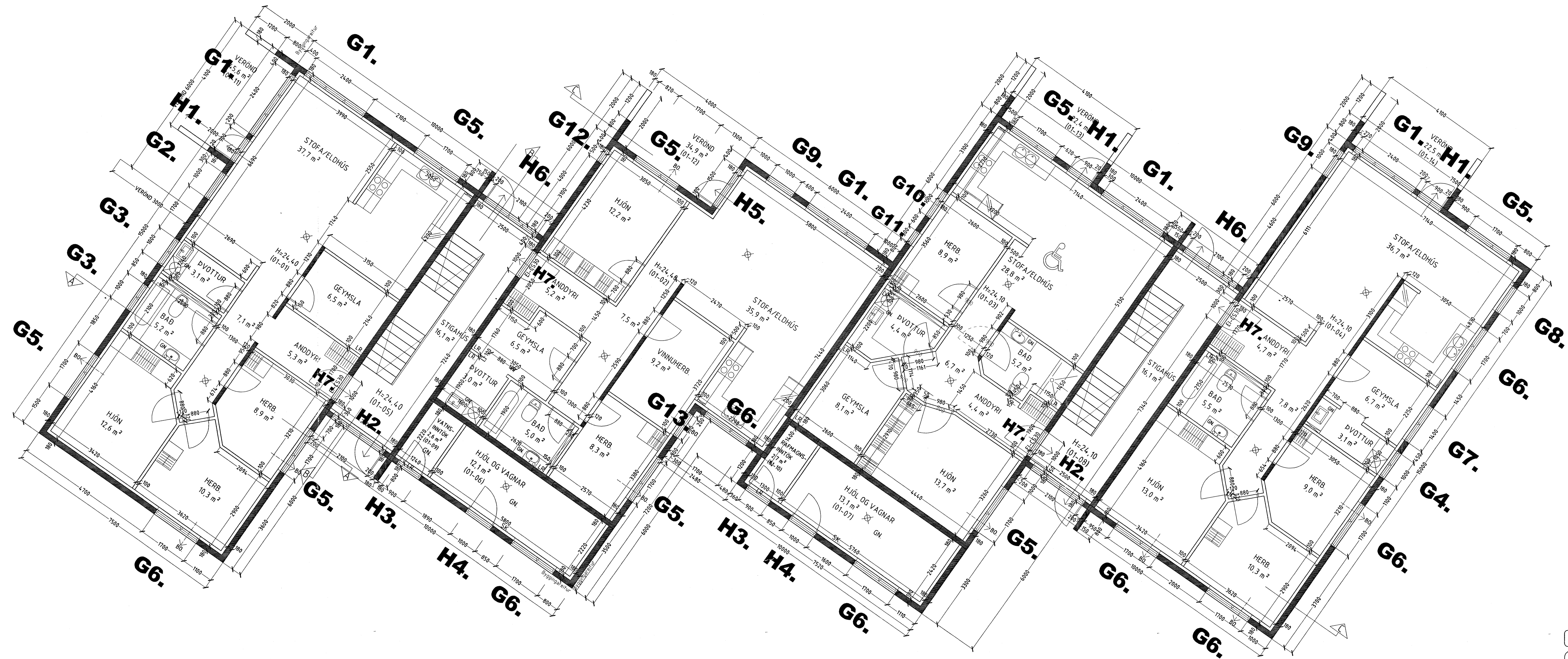
GRUNNMYND 1 HÆÐ. MKV. 1:50.
