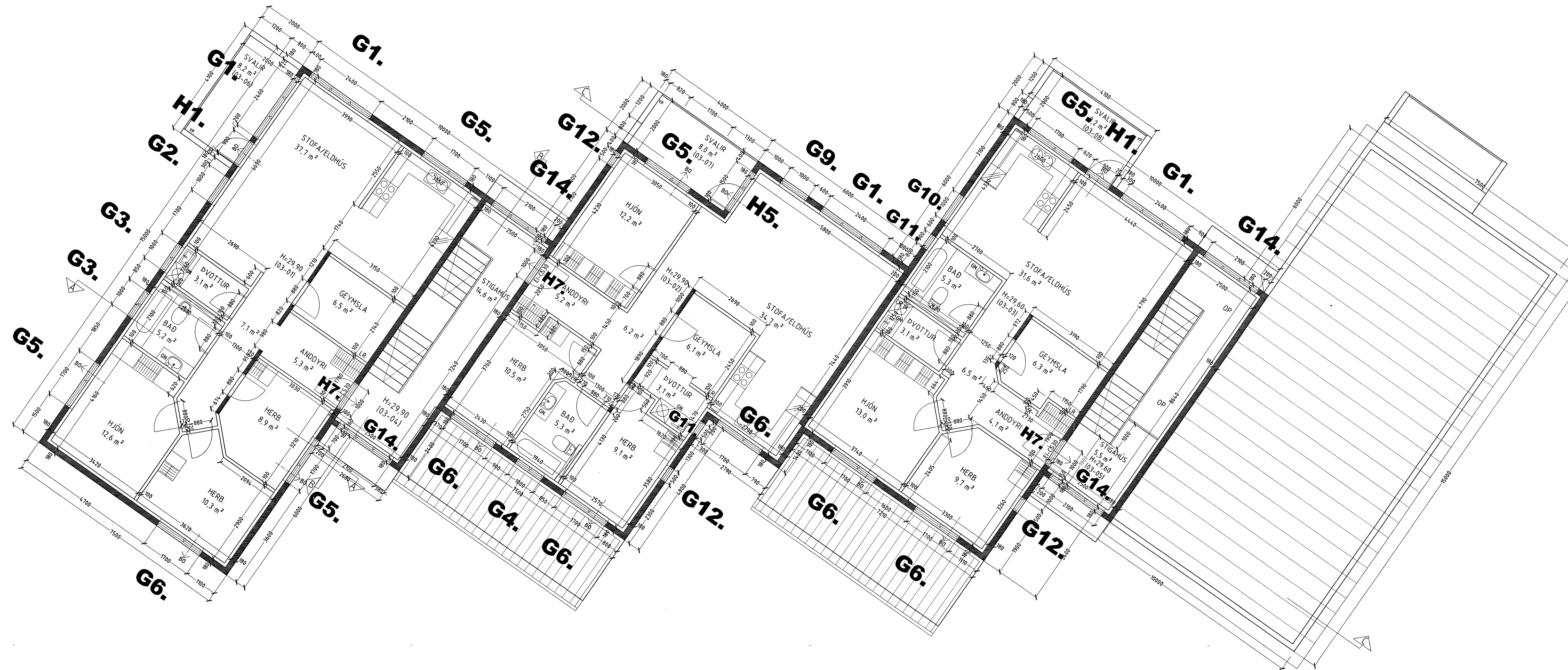
GRUNNMYND 3 HÆÐ. MKV. 1:50.
