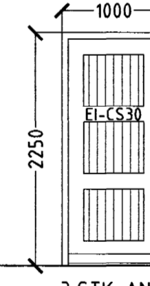
3 STK. ANDDYRI. HURÐ OPNAST HÆGRI INN.
