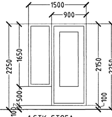
1 STK. STOFA. HURÐ OPNAST HÆGRI ÚT.
