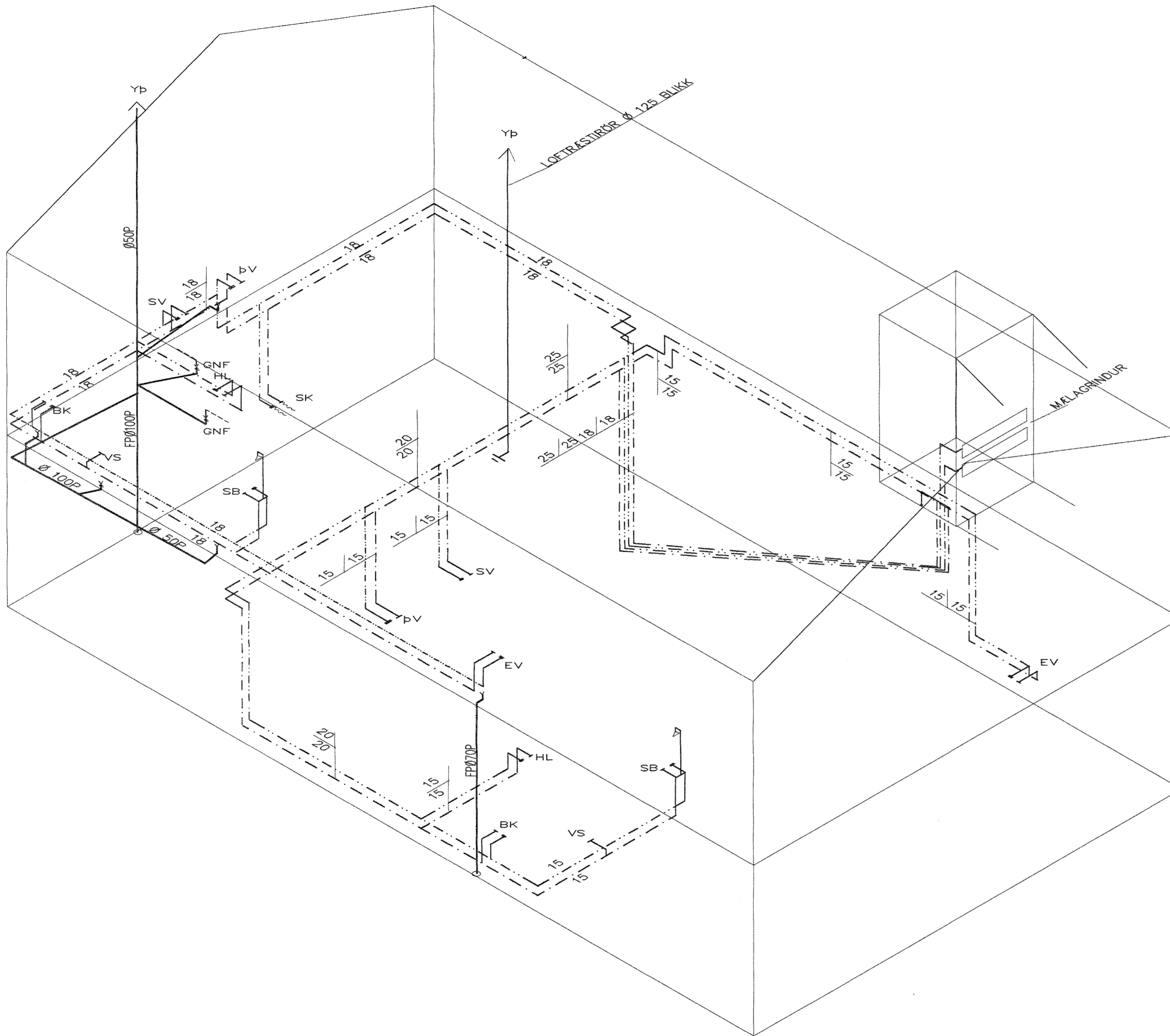
RÚMMYND VATNS OG FRÆRENNISLAGNA 1:50
