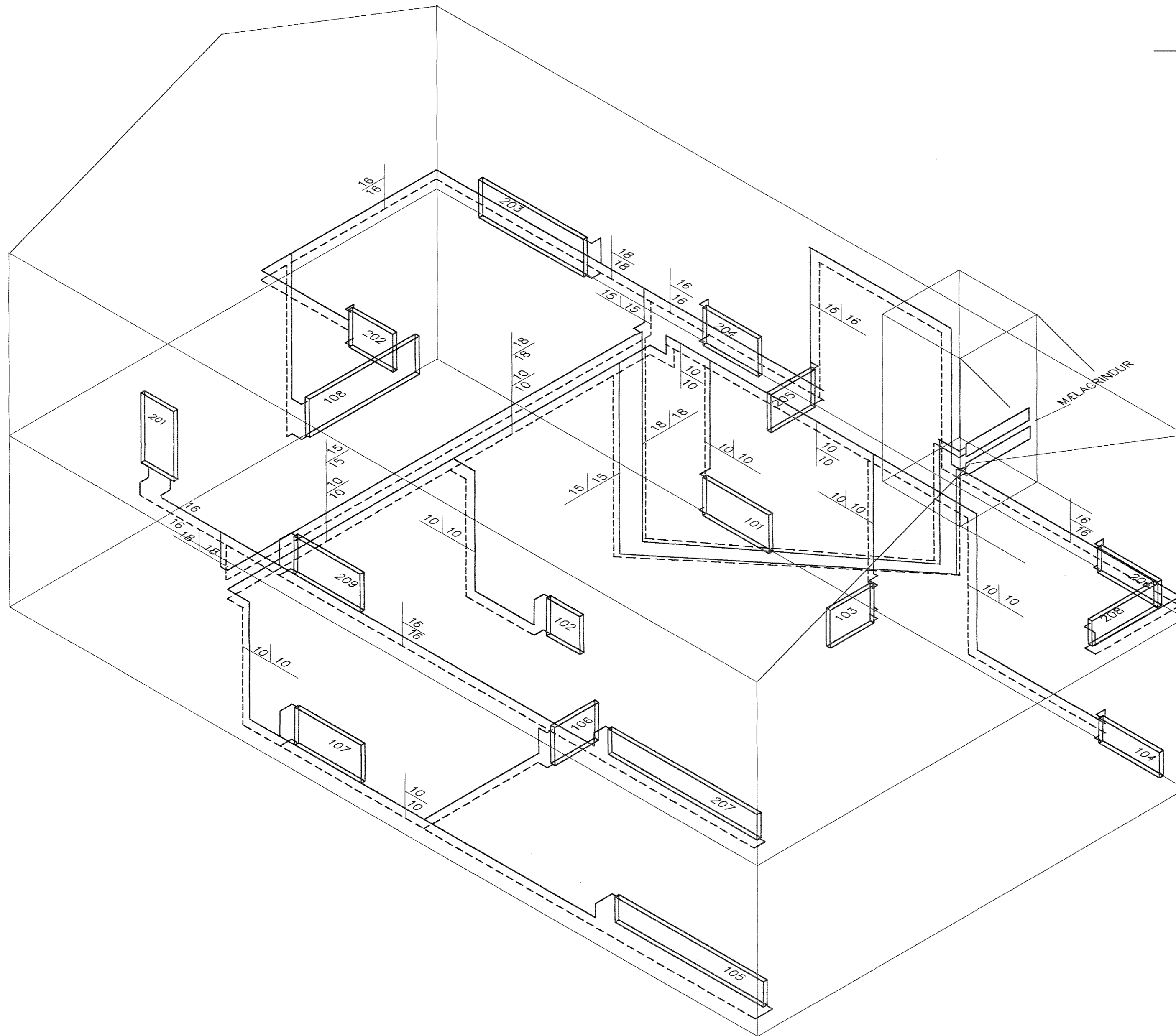
RÚMMYND HITALAGNA 1:50
