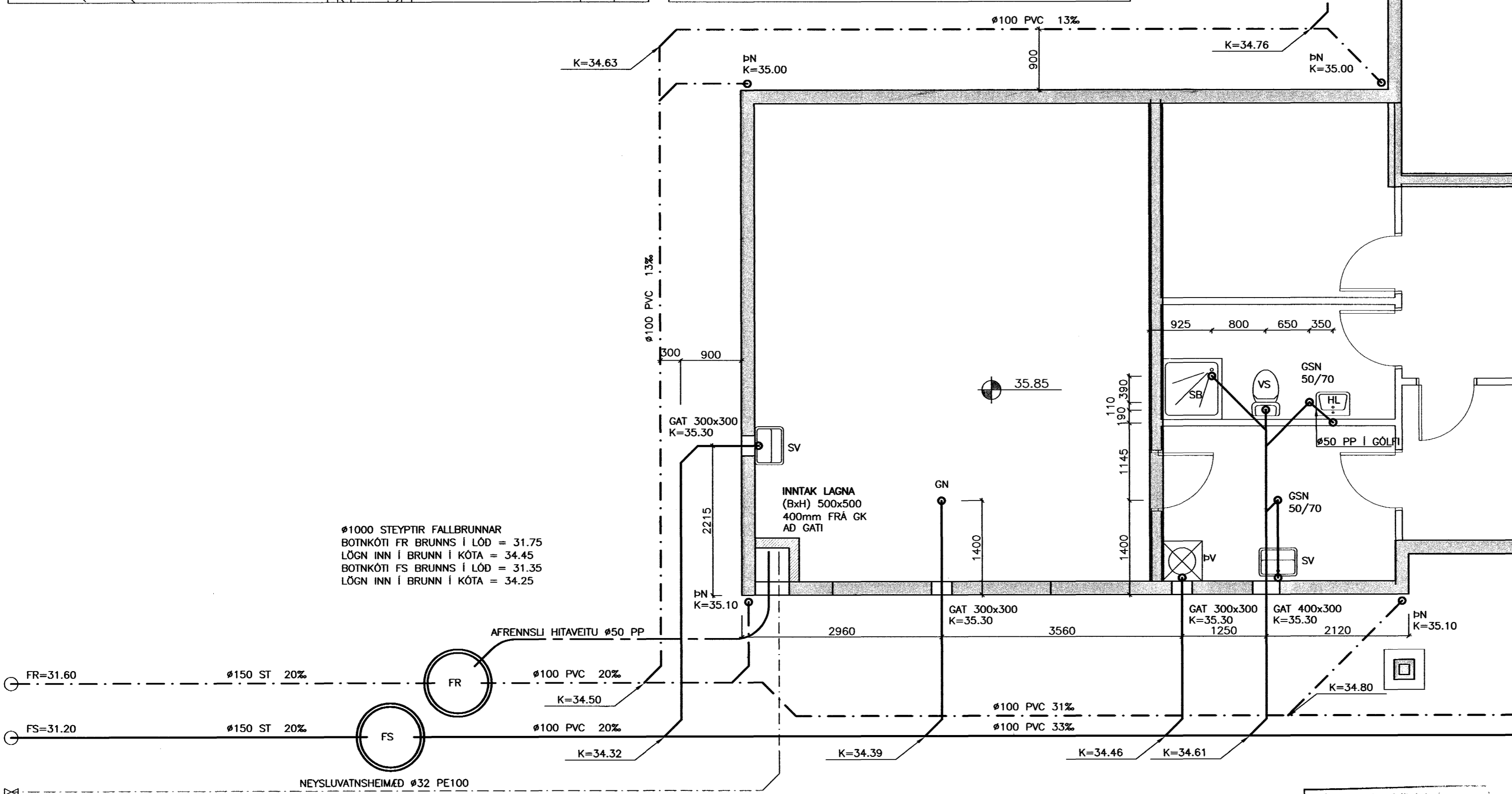
FALLBRUNNUR Mkv. 1:50
