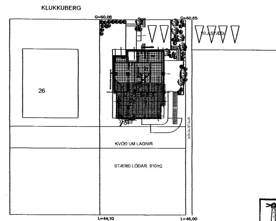
Afstöðumynd 1/500
