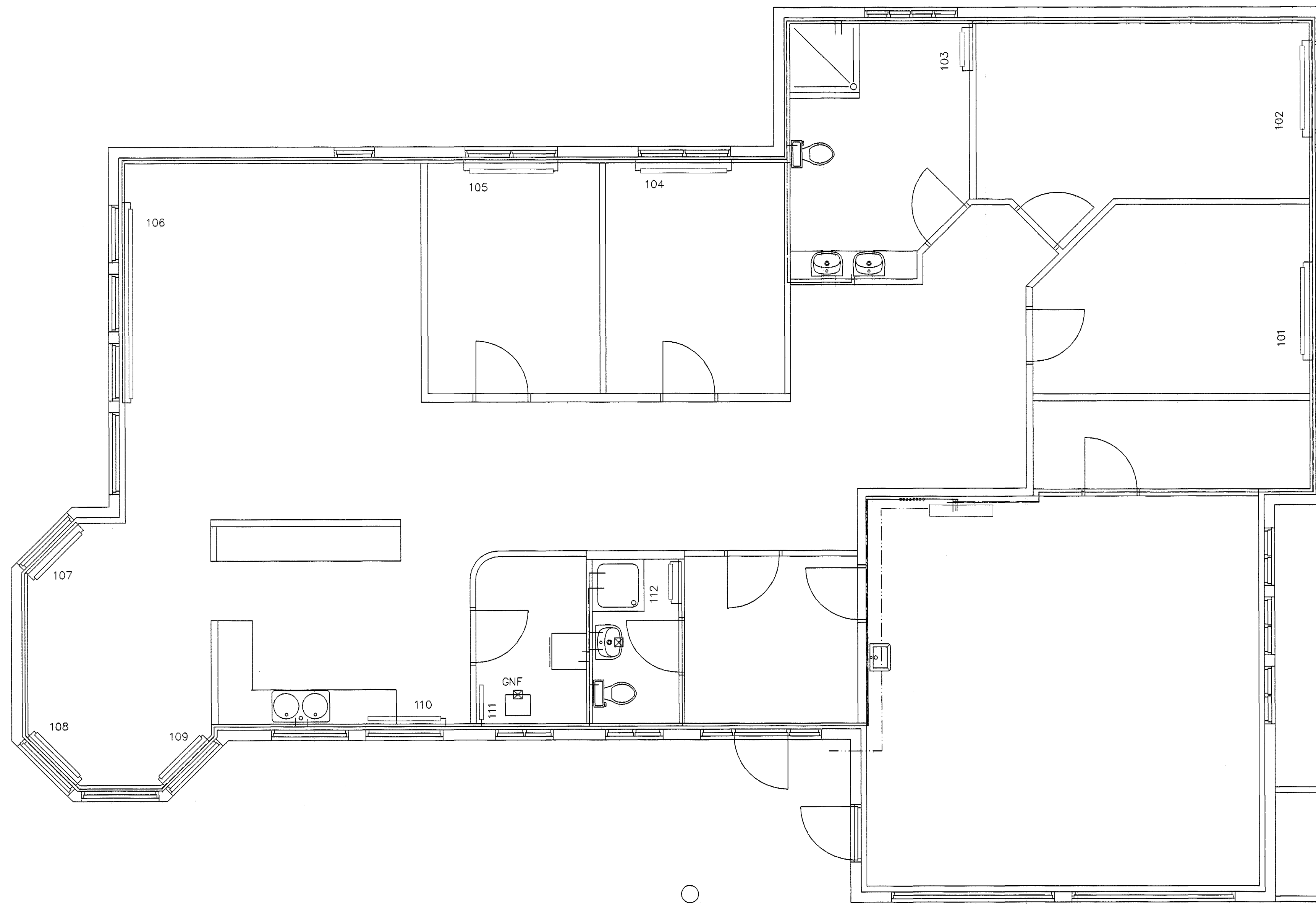
Grunnmynd 1/50
