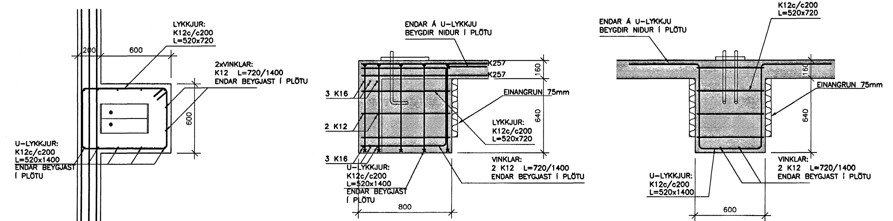
DEILI 1:20 B01/B02
