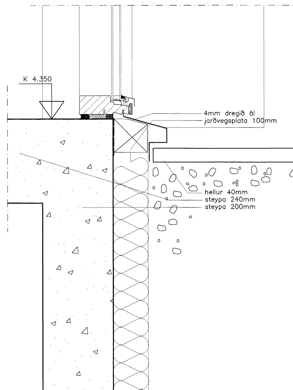
deili 16 / 23
