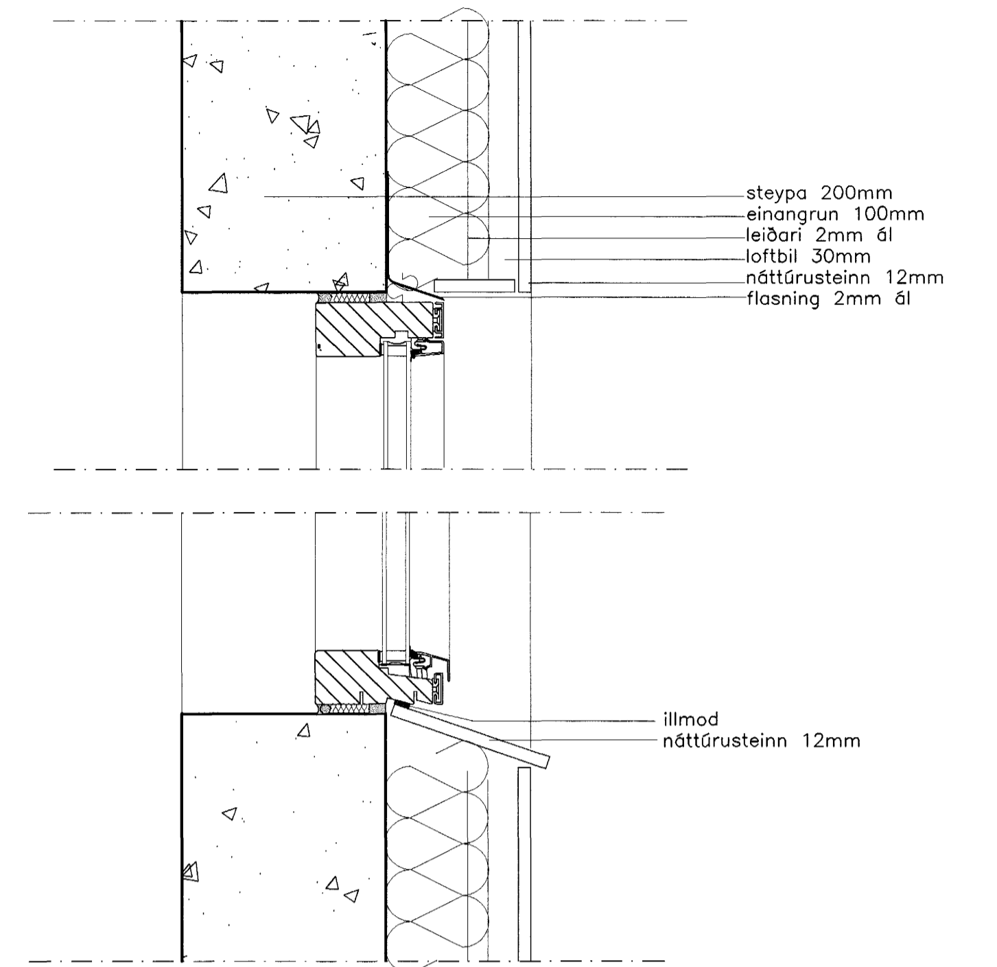
deili 17 / 10
