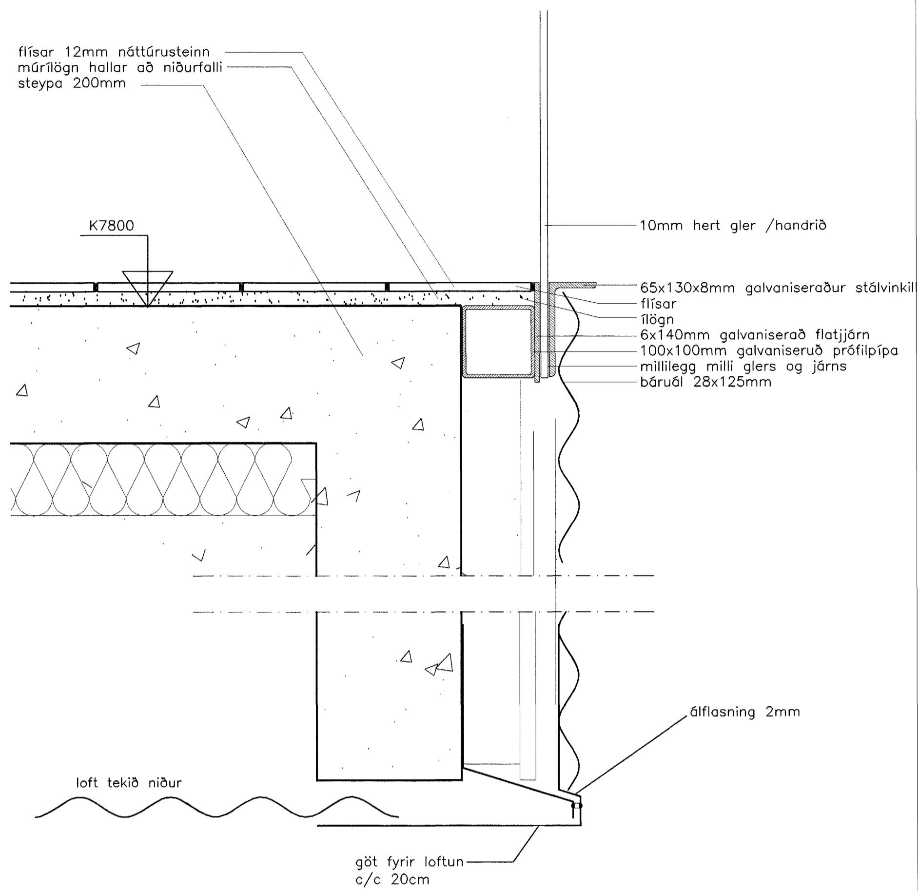
deili 13 / 22
