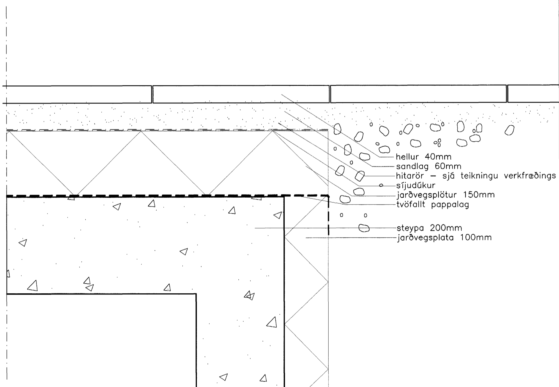
deili 14 / 22
