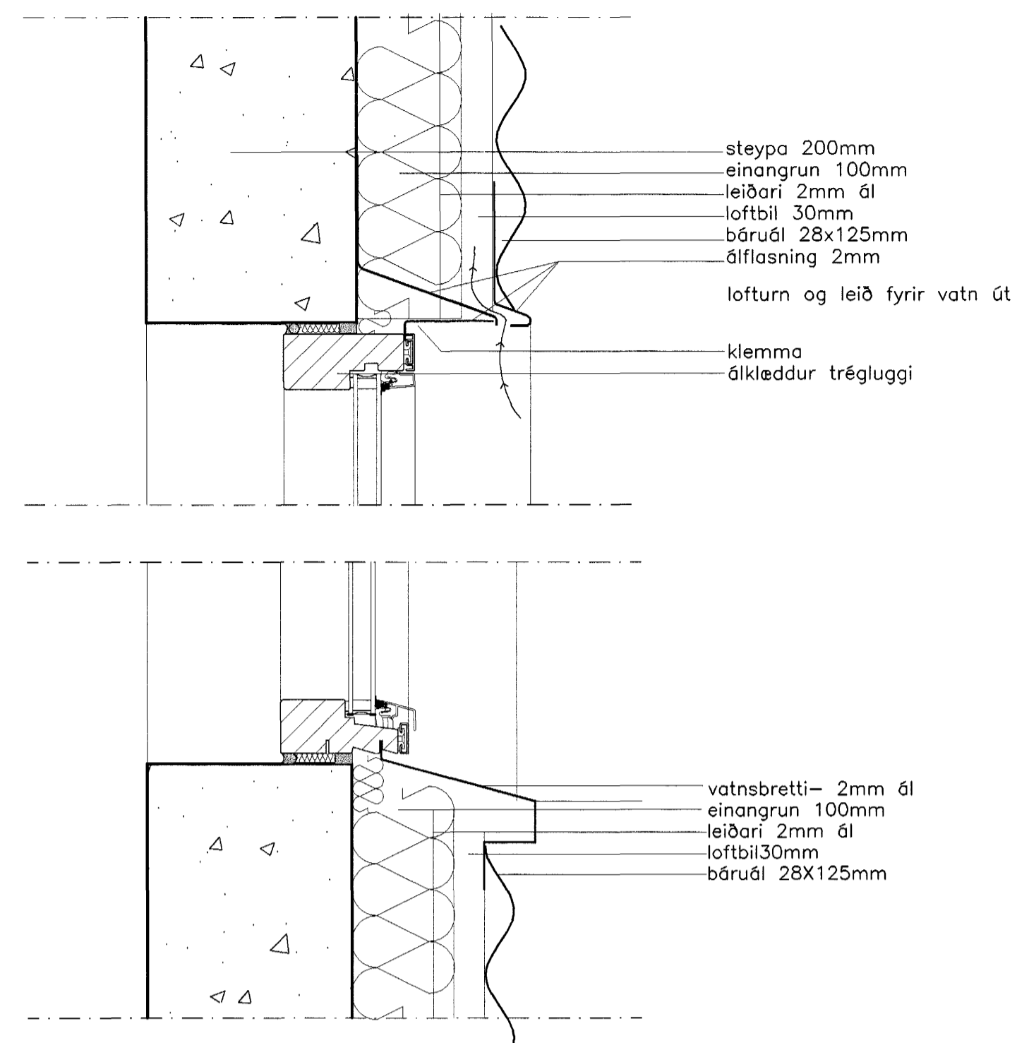
deili 15 / 23
