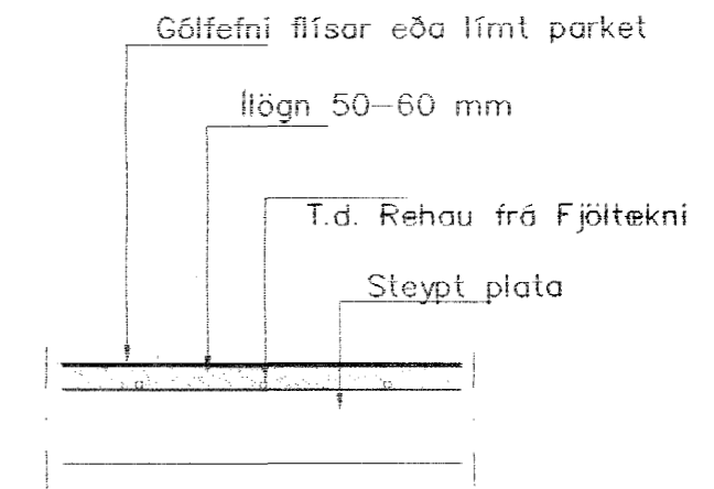
GÓLFHITALAGNIR SNIÐ 1:20
