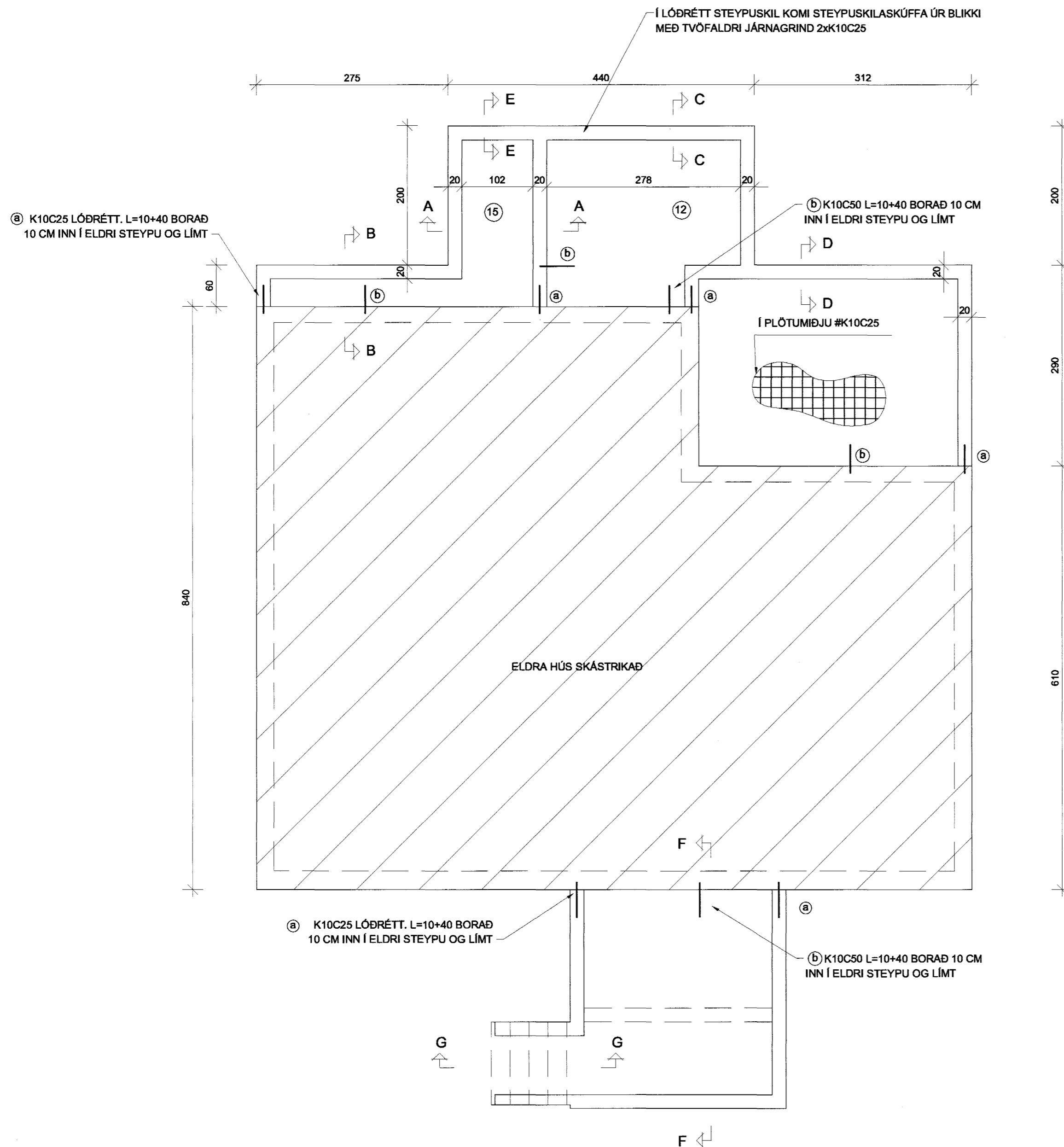
UNDIRSTÖÐUR, GRUNNMYND 1:50
