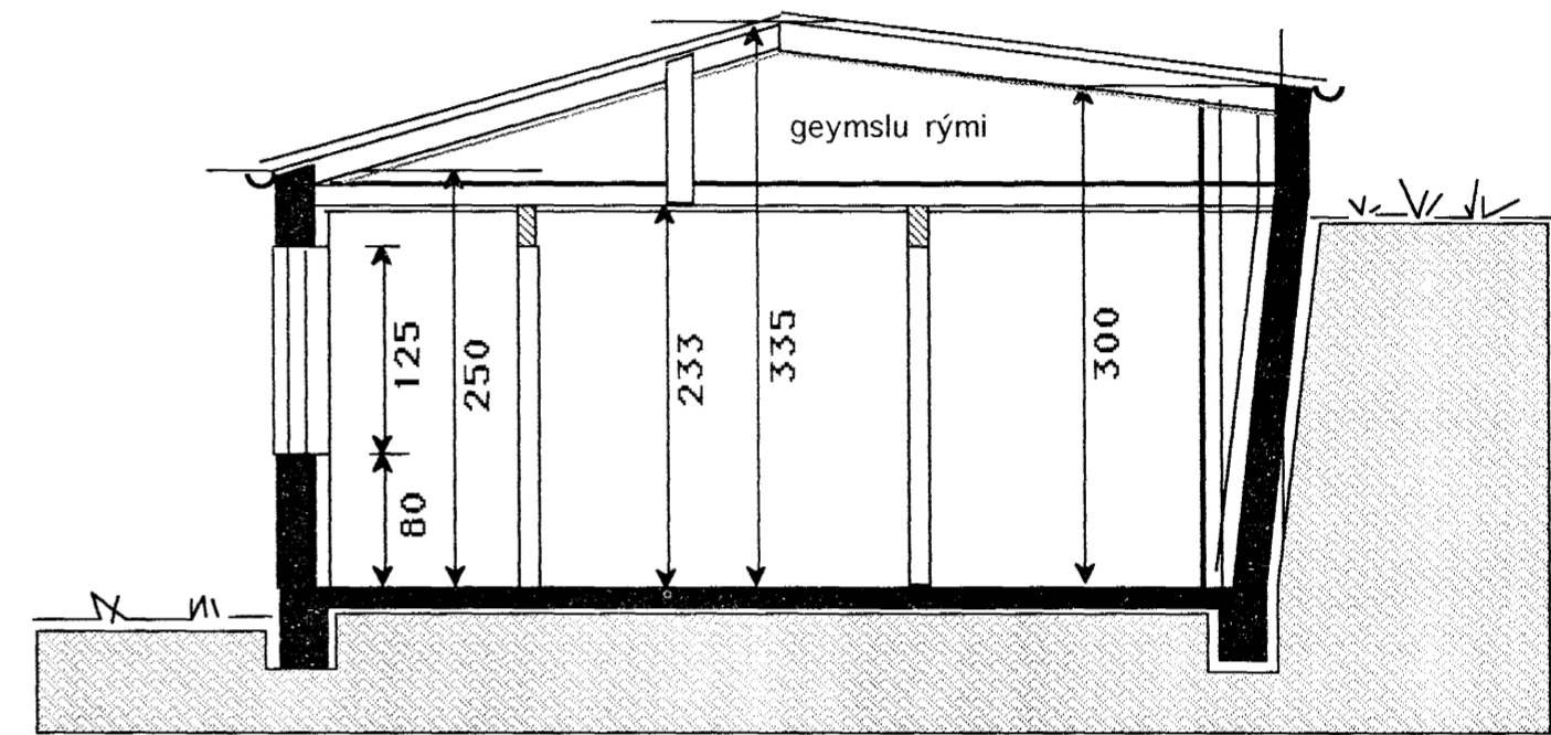
SNID A-A
