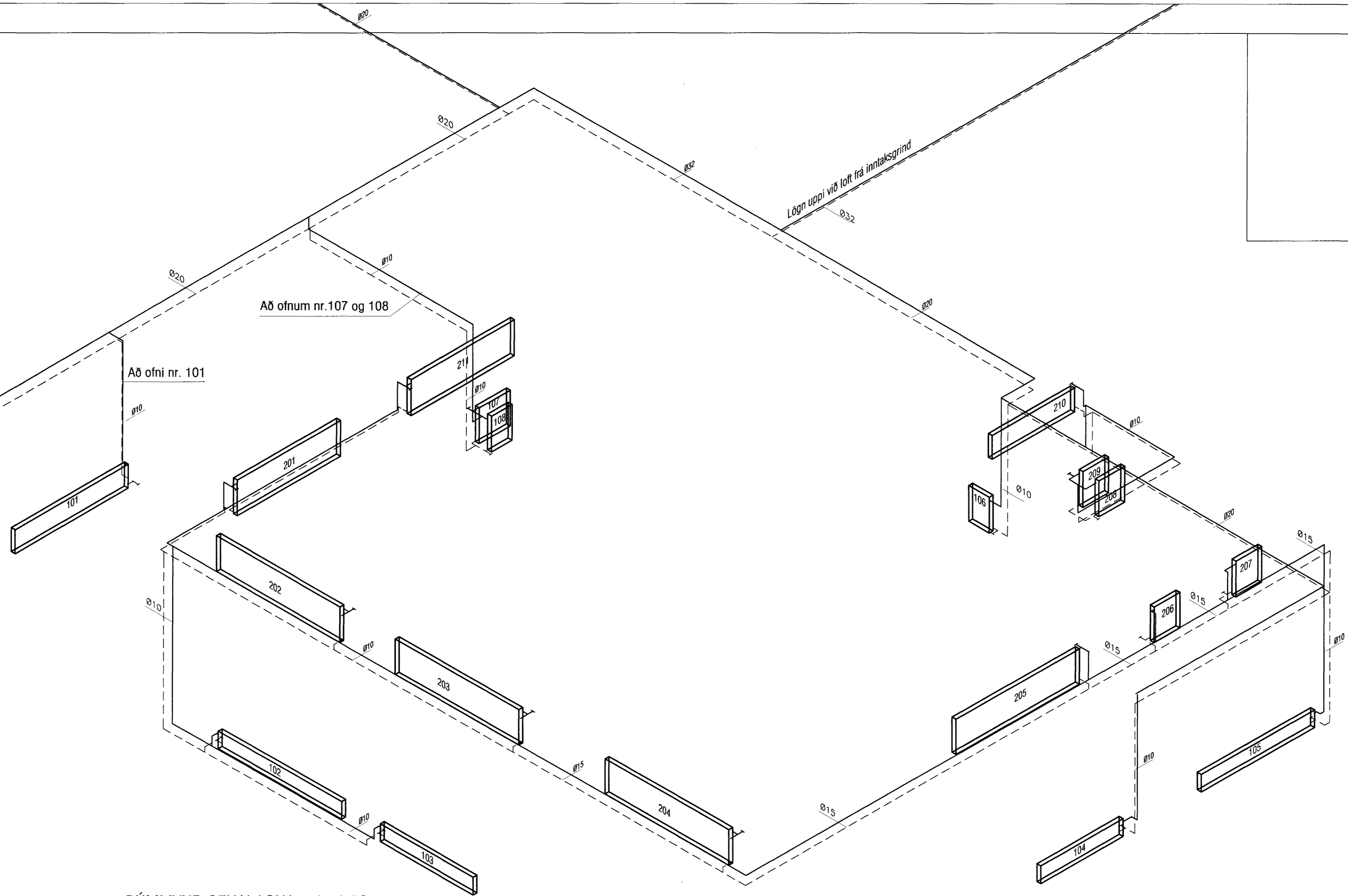
RÚMMYND OFNALAGNA mkv.1:50
