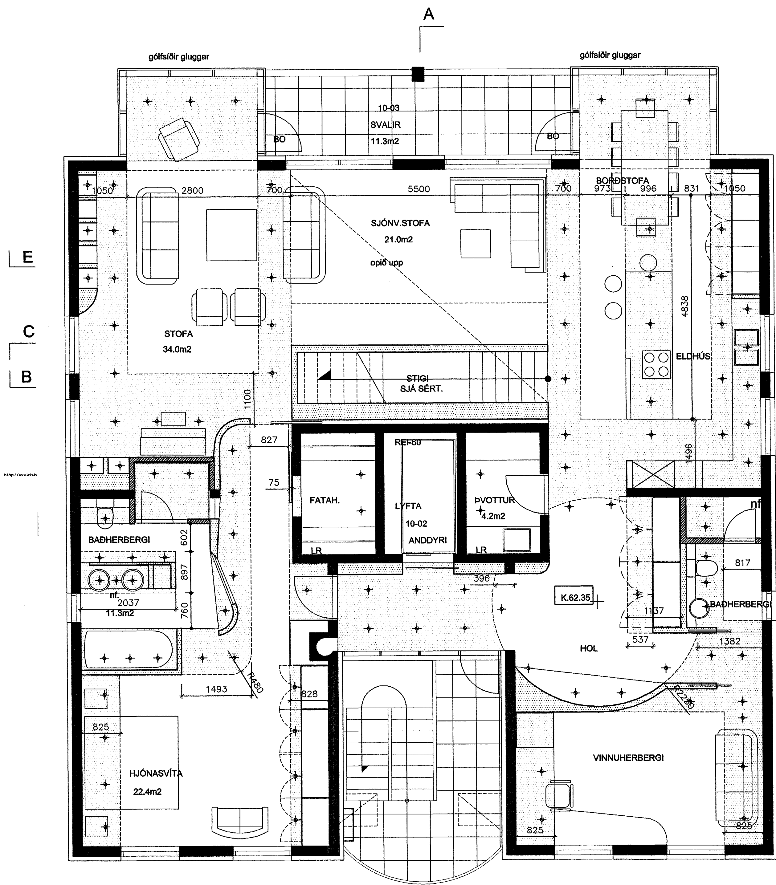
GRUNNMYND 10.HÆÐ mkv.1.50 YFIRLIT NIÐURTEKIN GIFSLOFT INNFELLD HALOGENLÝSING NÁNARI ÚTFÆRSLA SJÁ SÉRTEIKNINGAR 1.20 OG ÁSÝNDIR.
