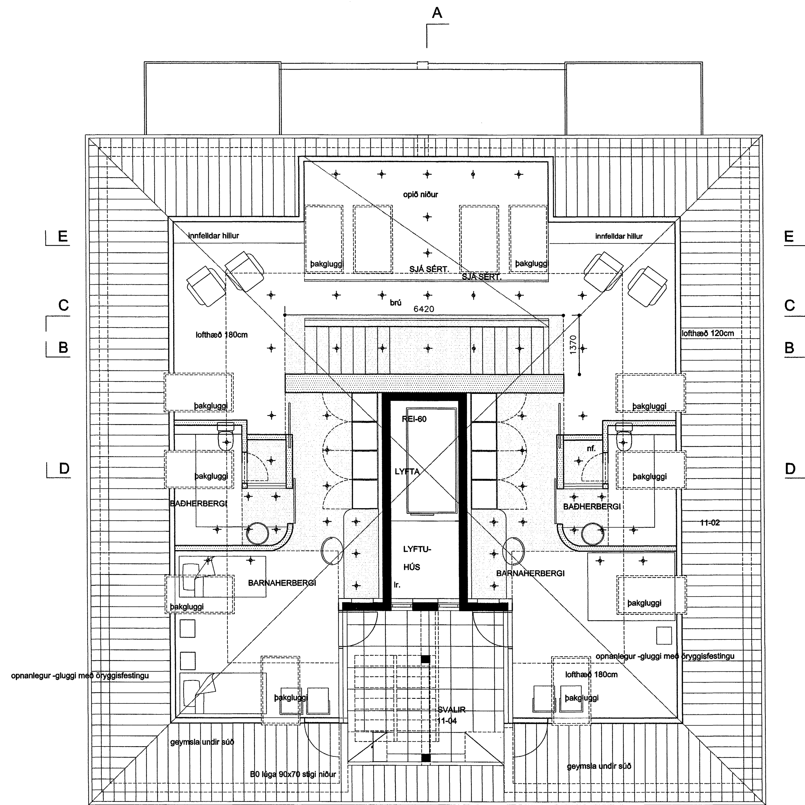
GRUNNMYND RISHÆÐ mkv.1.100 YFIRLIT NIÐURTEKIN GIFSLOFT INNFELLD HALOGENLÝSING NÁNARI ÚTFÆRSLA SJÁ SÉRTEIKNINGAR 1.20 OG ÁSÝNDIR.
