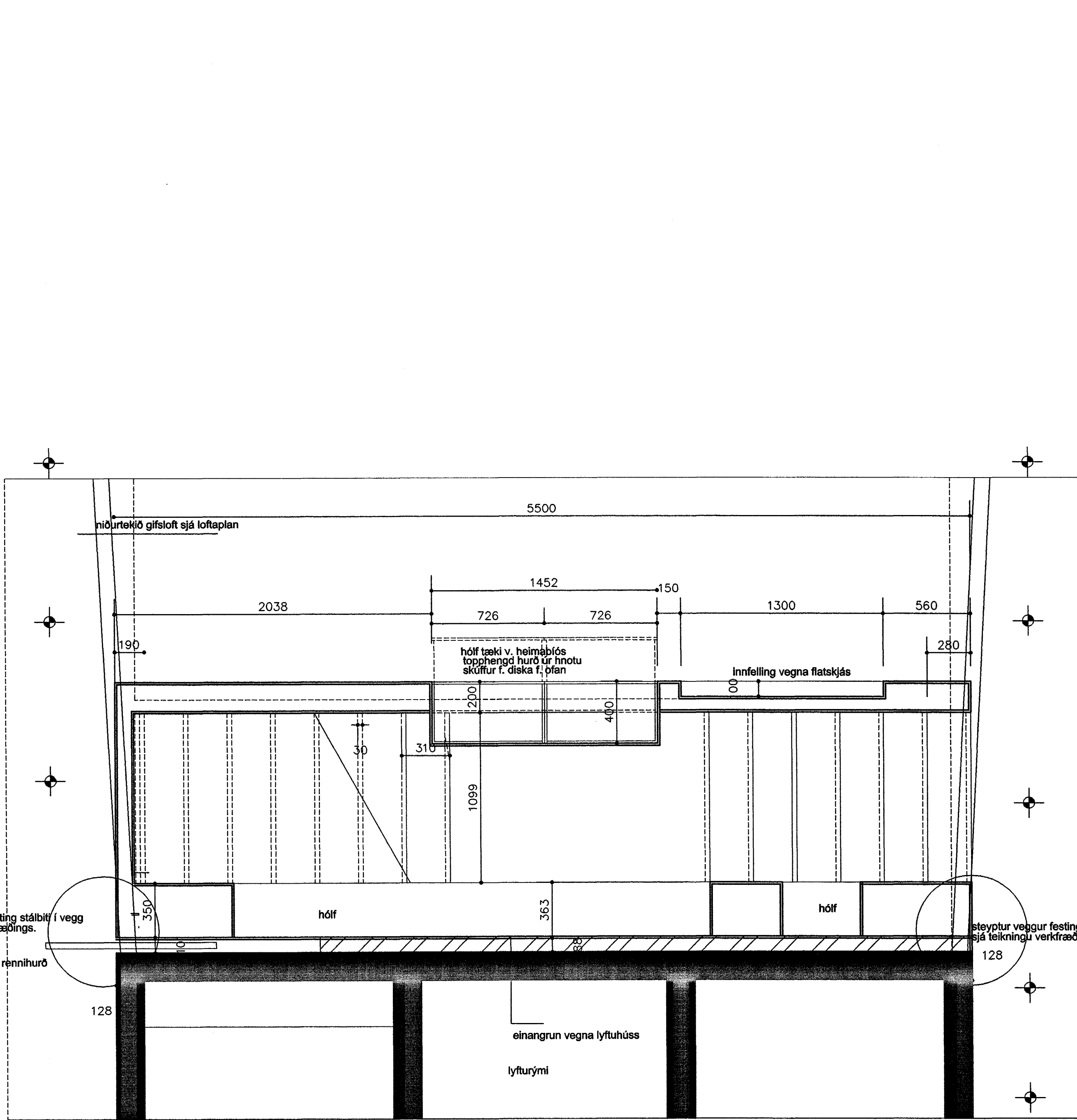
GRUNNMYND STIGI mkv.1.20
