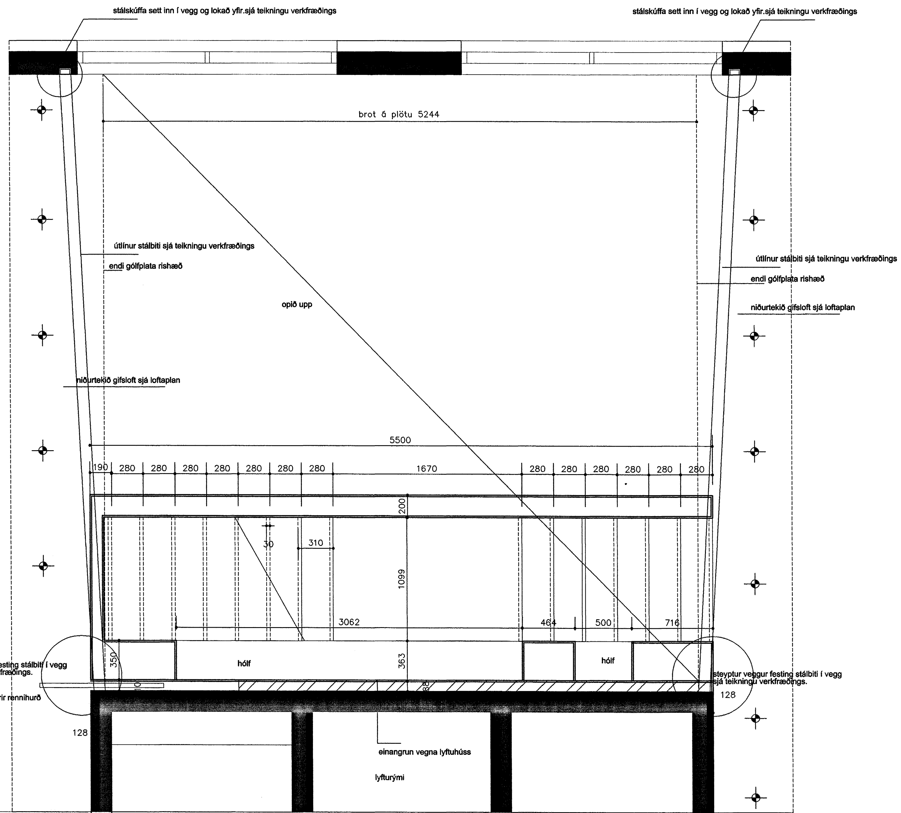
GRUNNMYND STIGI mkv.1.20
