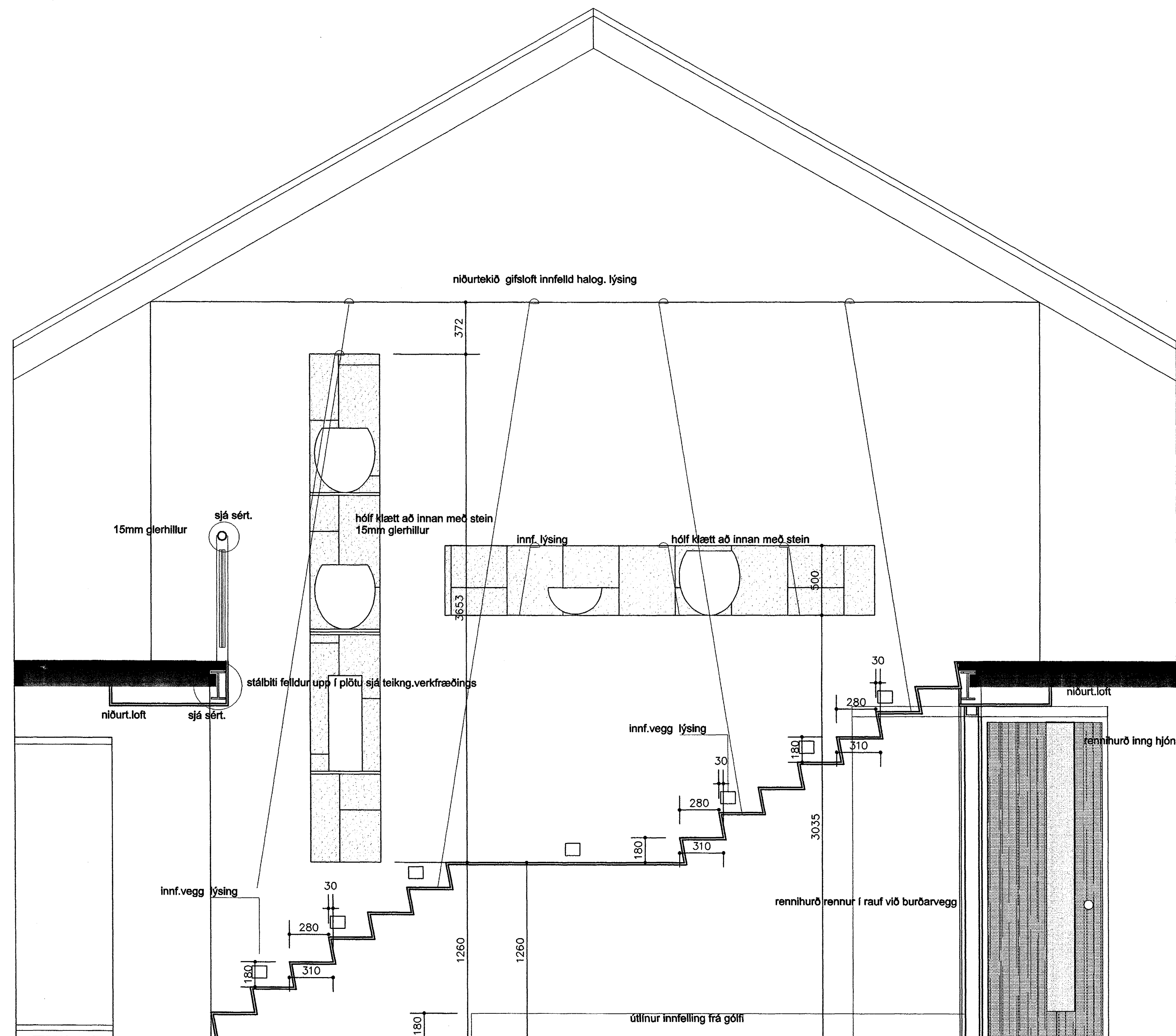
ÁSÝND SNÍÐMYND STIGI mkv.1.20
