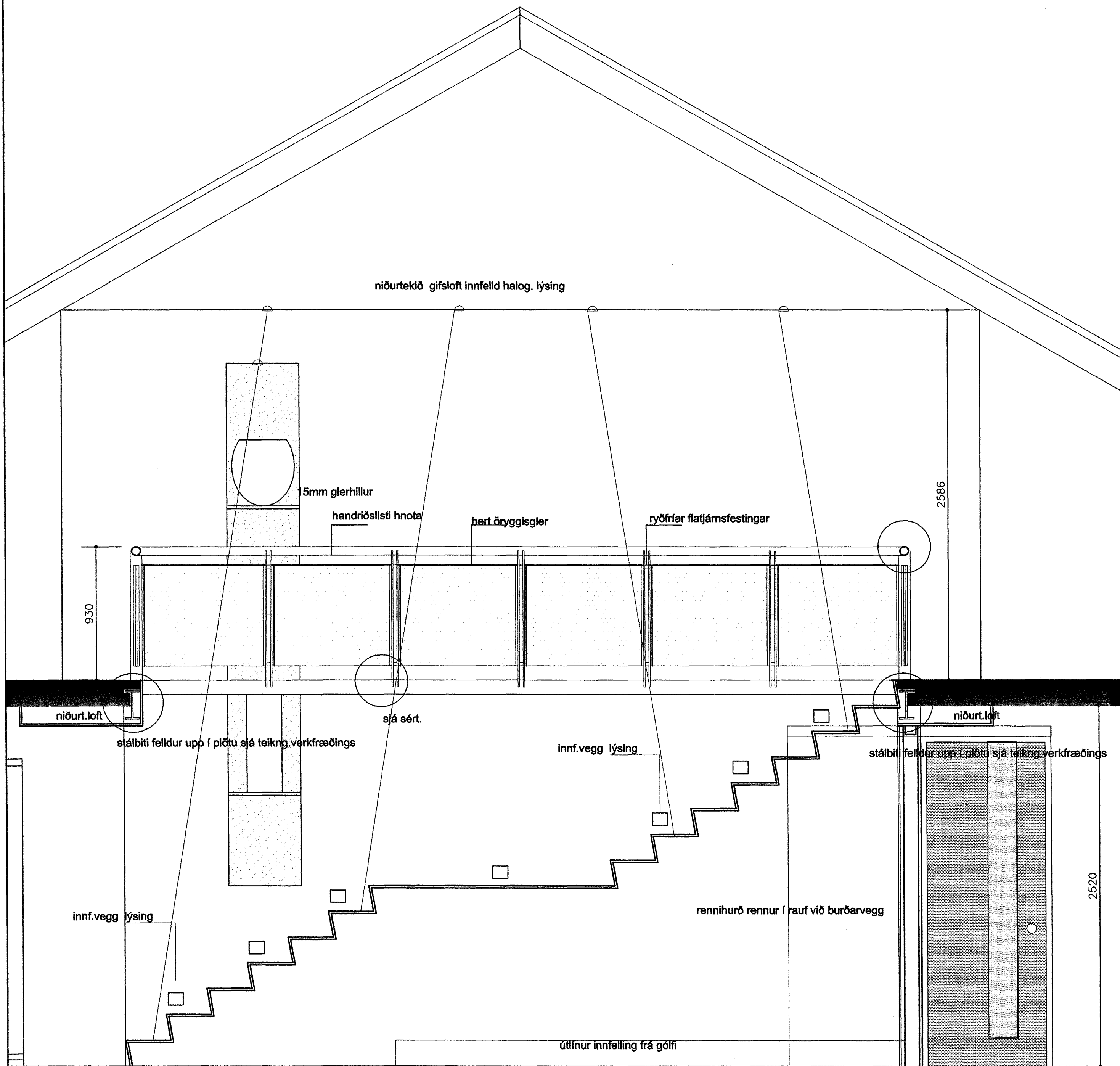
SNÍÐMYND STIGI mkv.1.20
