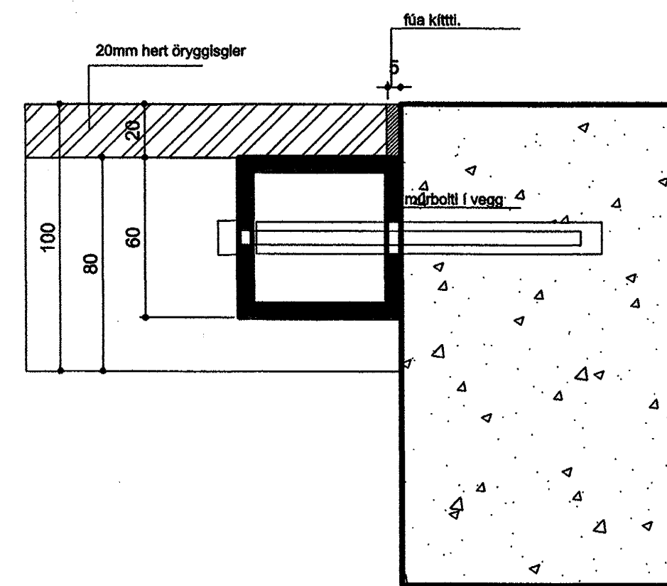
FESTINGAR FRÁGANGUR VIÐ ENDA mkv.1.2
