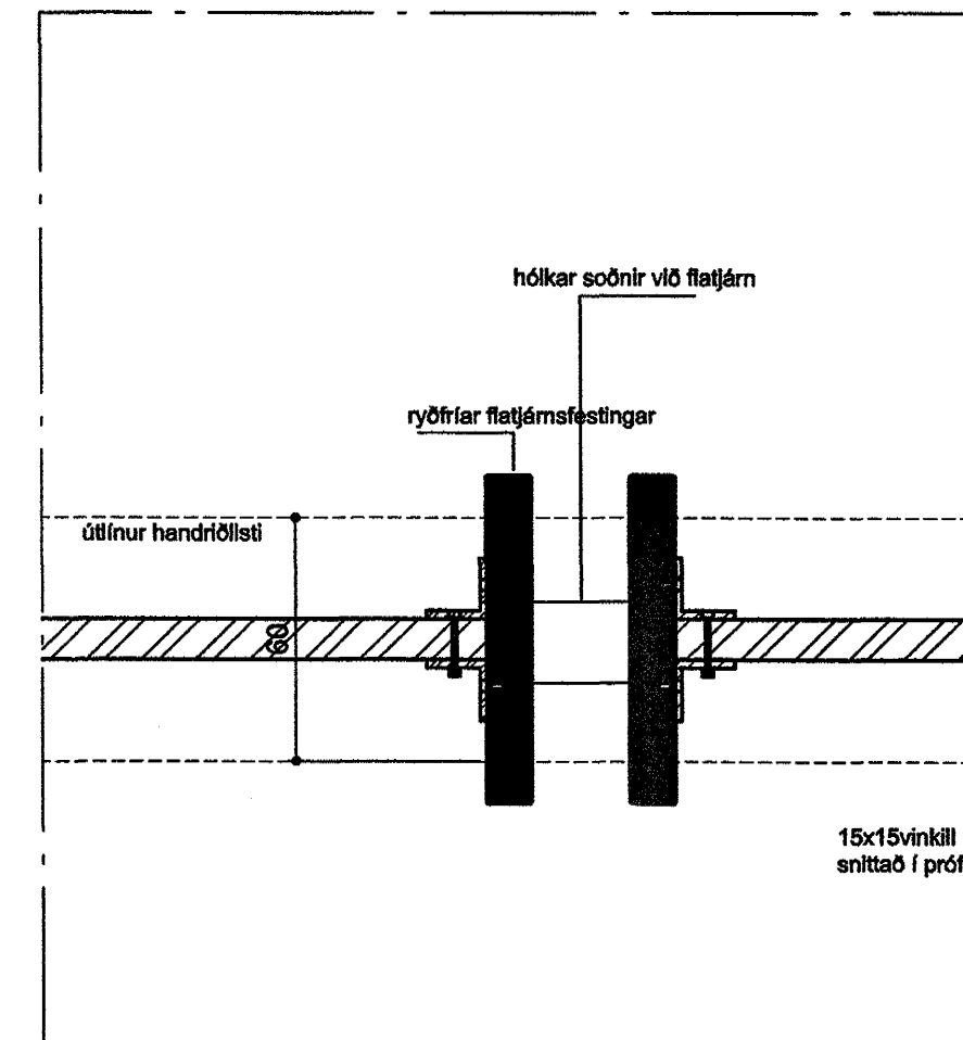
LÁRÉTT SNIÐ Í HANDRÍÐ mkv.1.2
