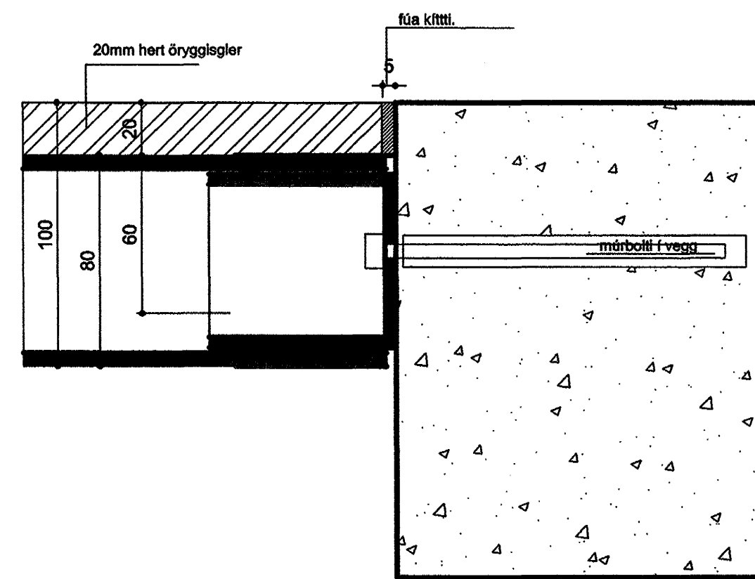
FESTINGAR FRÁGANGUR VIÐ ENDA mkv.1.2
