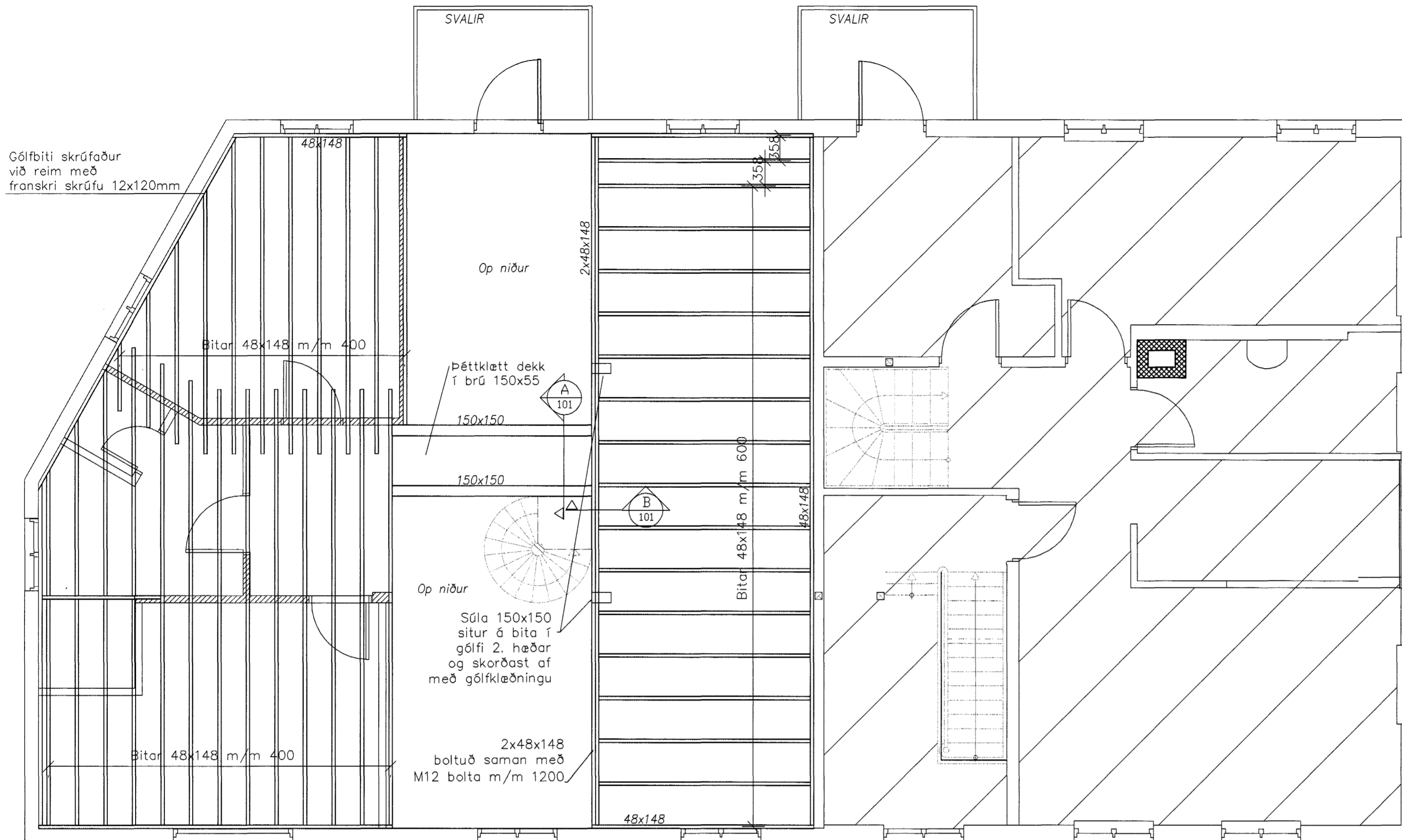
Grunnmynd 2.hæð Mælikvarði 1:50
