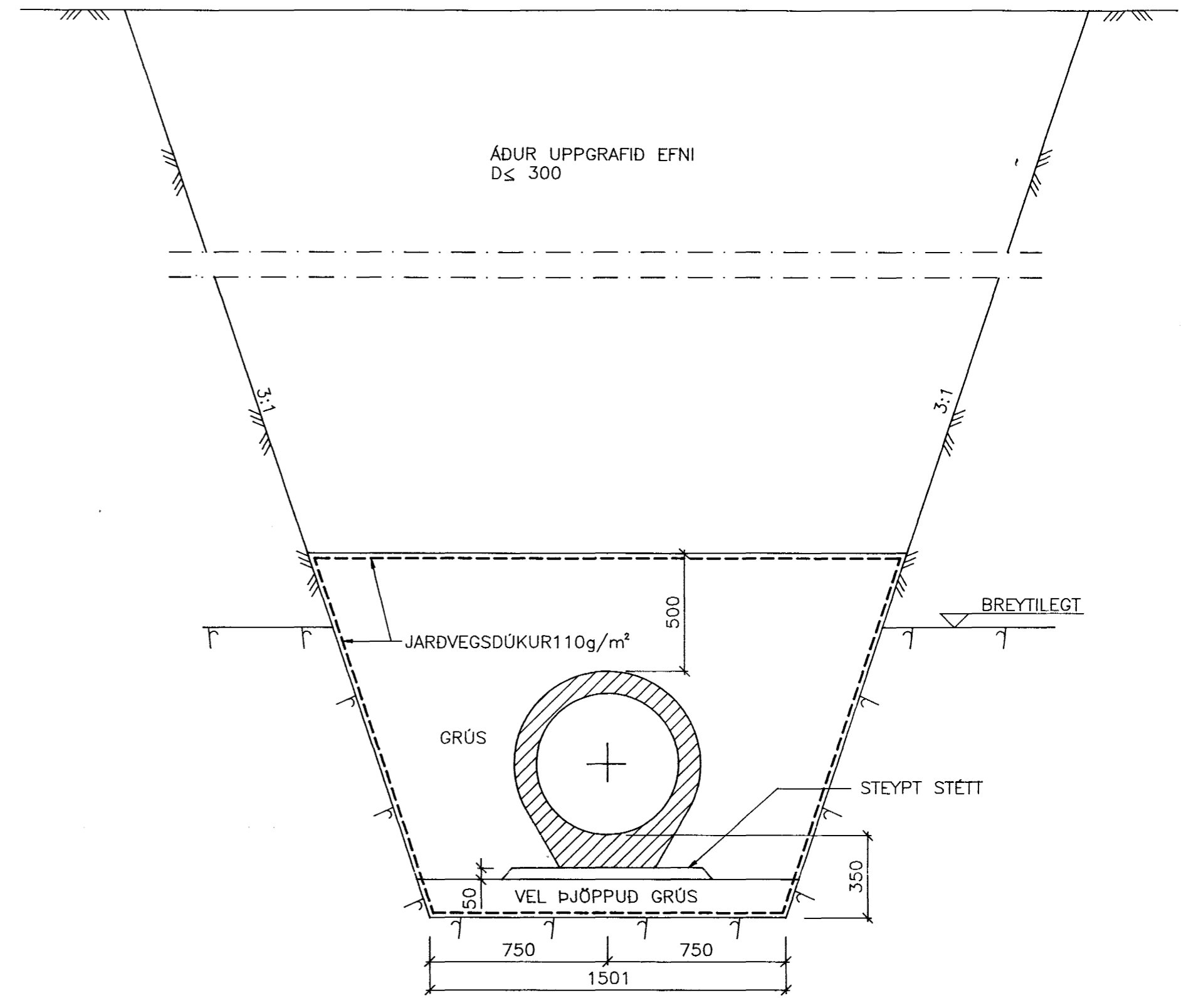
ÞVERSNIÐ Í LAGNASKURÐ 1:20
