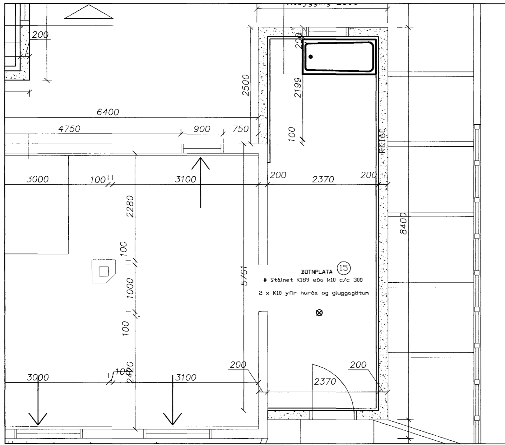
GRUNNMYND STEYPRA VEGGJA MKV. 1:50
