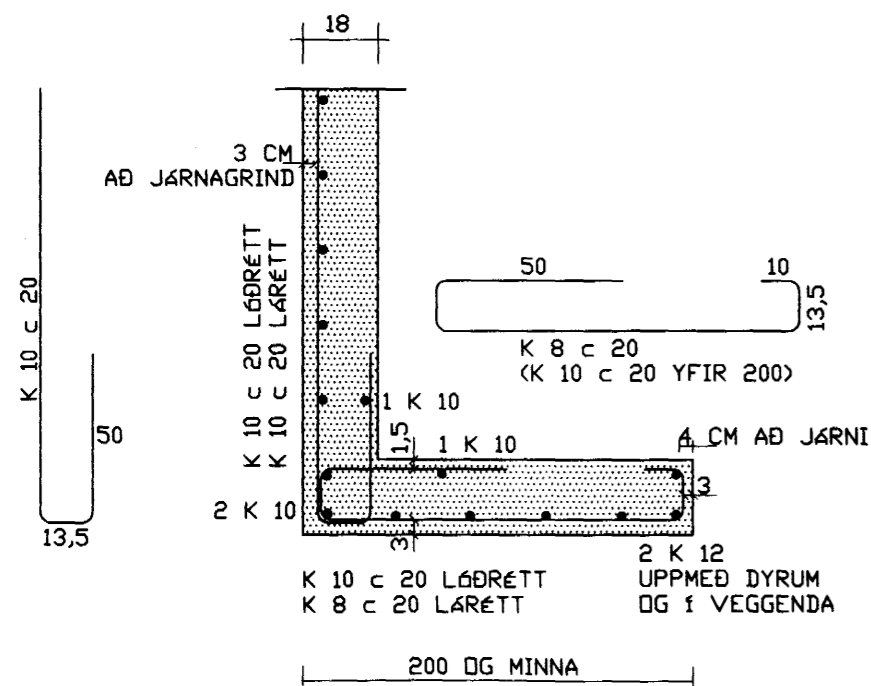
JÁRN Í ÖTVEGGI HÆÐA, LÁRÉTT SNIÐ Í ÖTHORN 1:20
