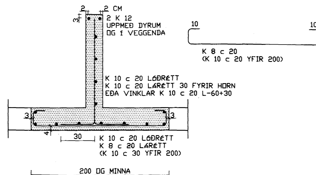
JÁRN Í INNVEGGI HÆÐA, LÁRÉTT SNIÐ Í ÖT- OG INNVEGG MILLI GLUGGA 1:20
