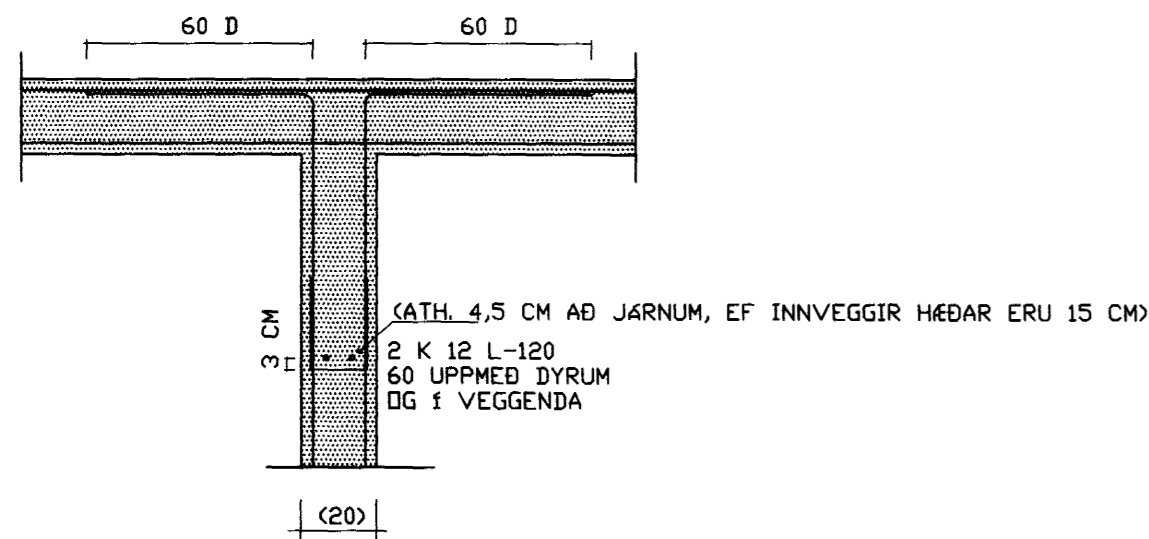
JÁRN Í UNDIRSTÖÐUR, LÁRÉTT SNIÐ Í ÖTVEGG VIÐ INNVEGG 1:20
