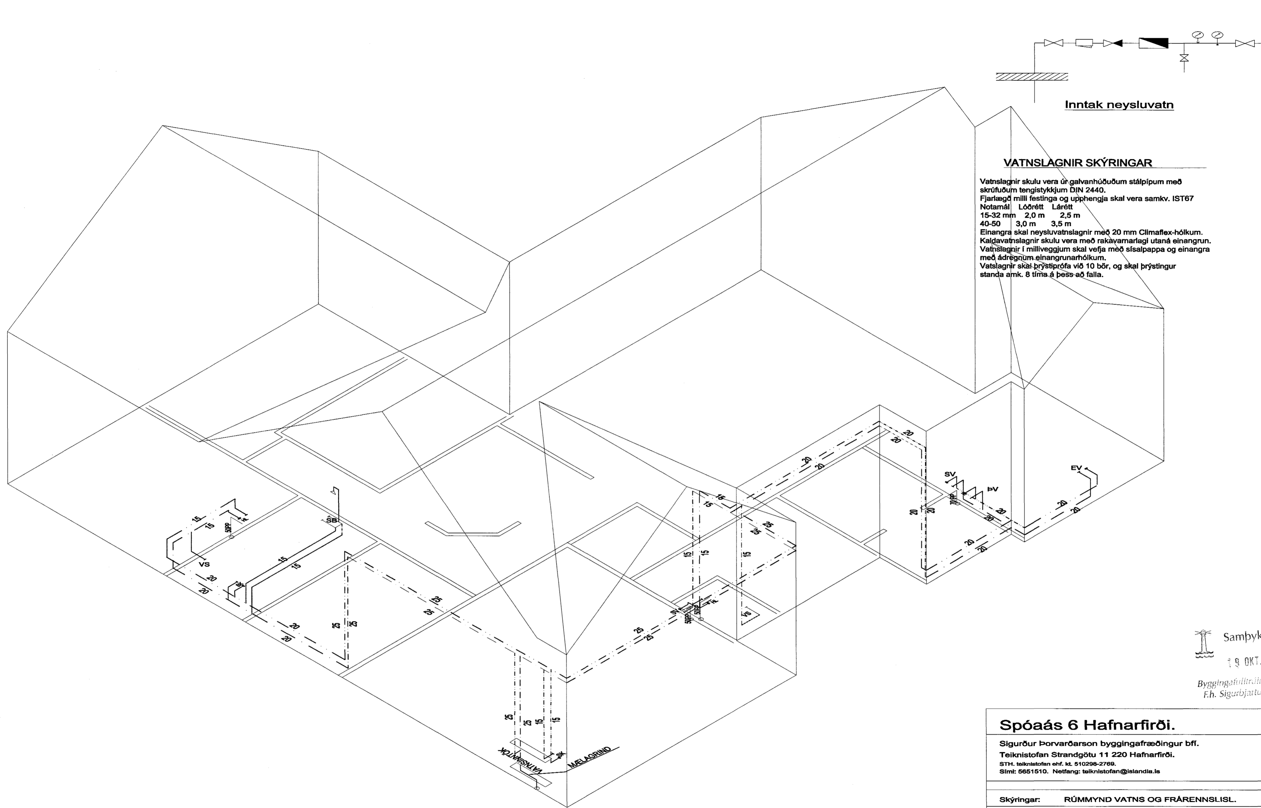
RÚMMYND VATNS OG FRÁRENNSLISLAGNA 1:50
