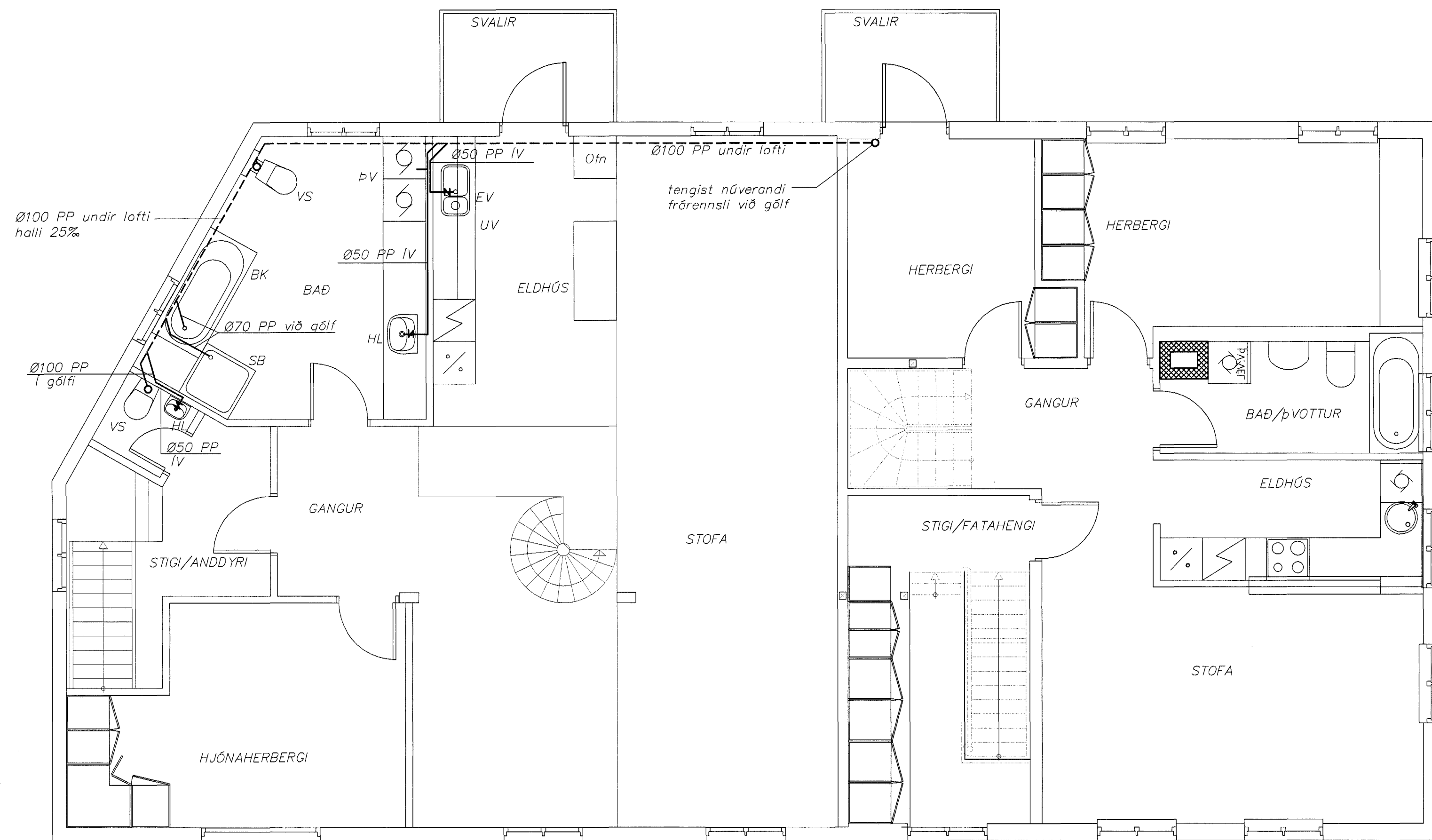
Grunnmynd 2. hæð
