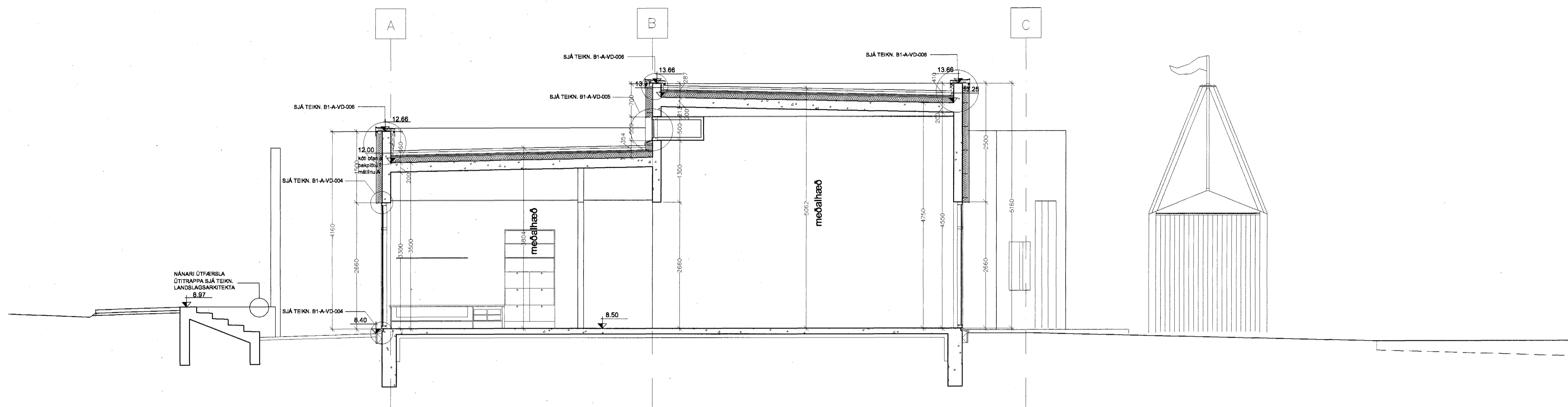
ÞVERSNIÐ A:A
