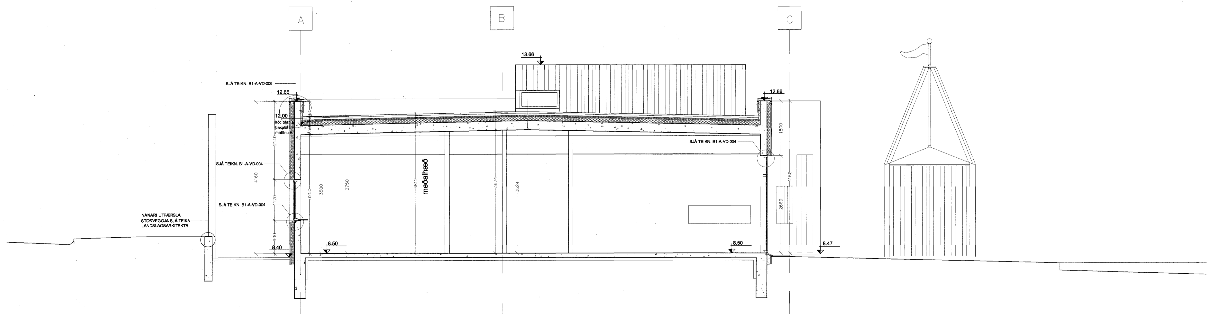
ÞVERSNIÐ B:B
