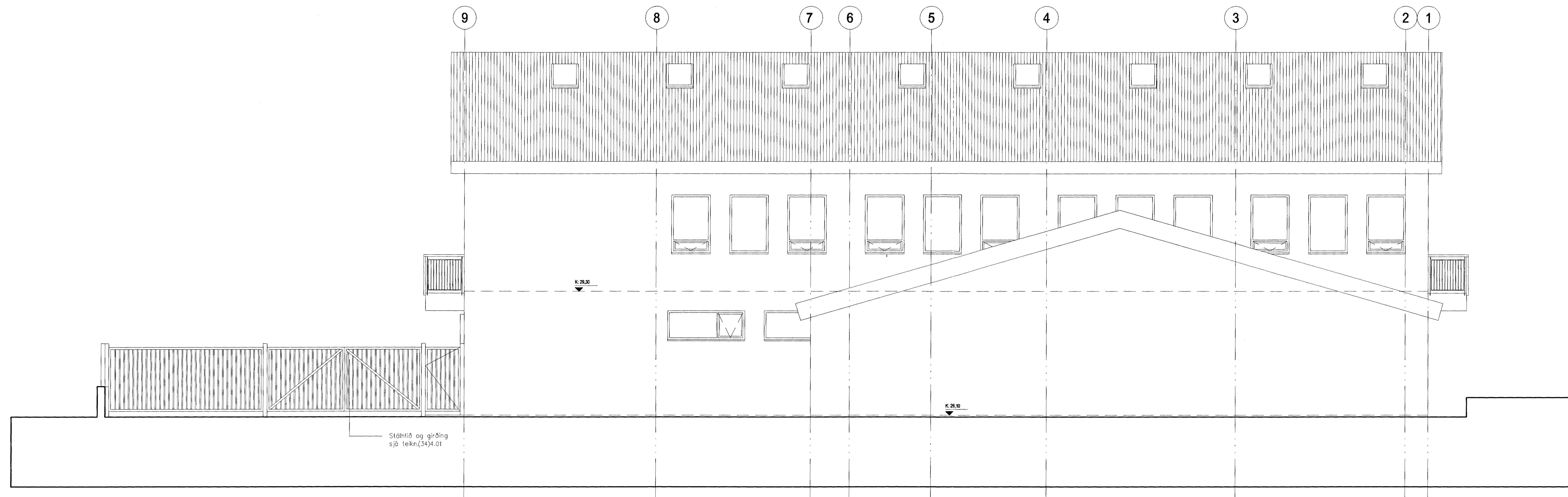
Austur útlit mkv.: 1:50
