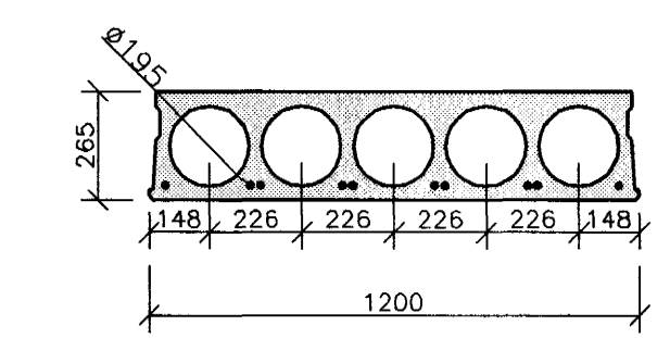
SNID I HP265 1:20
