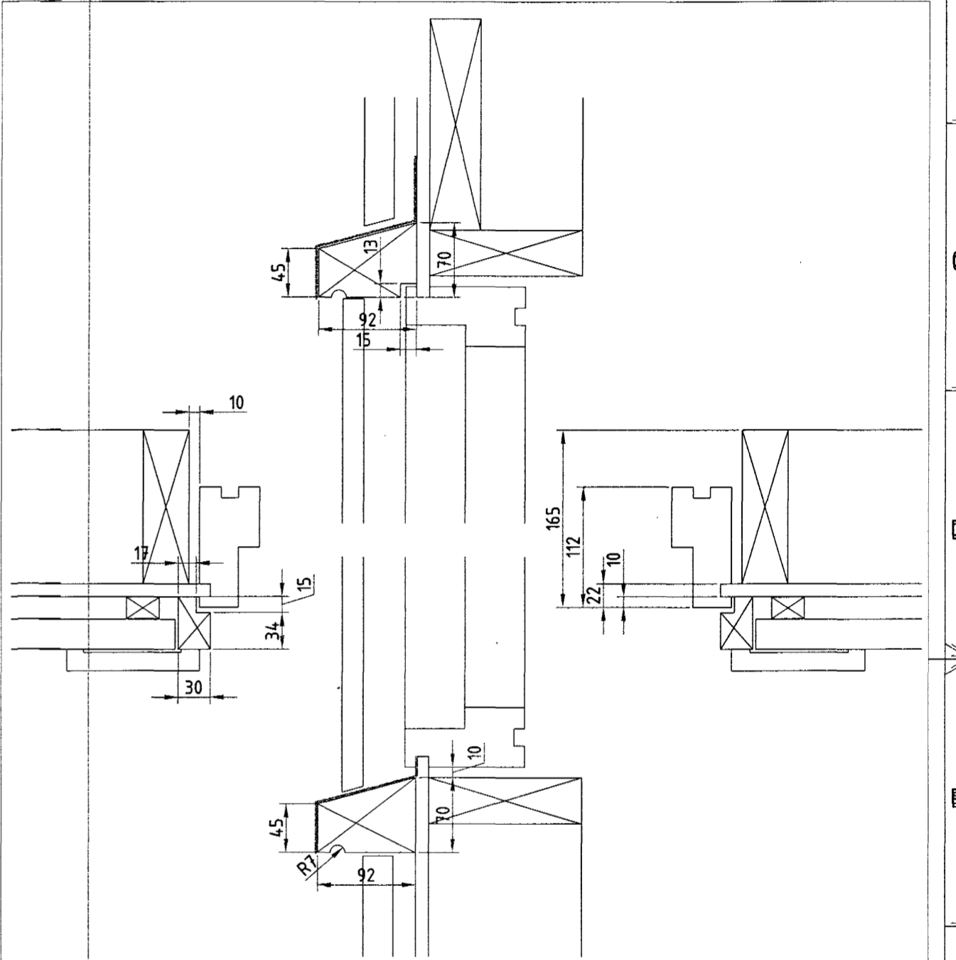
Frágangur kringum glugga.Mk 1:5.
