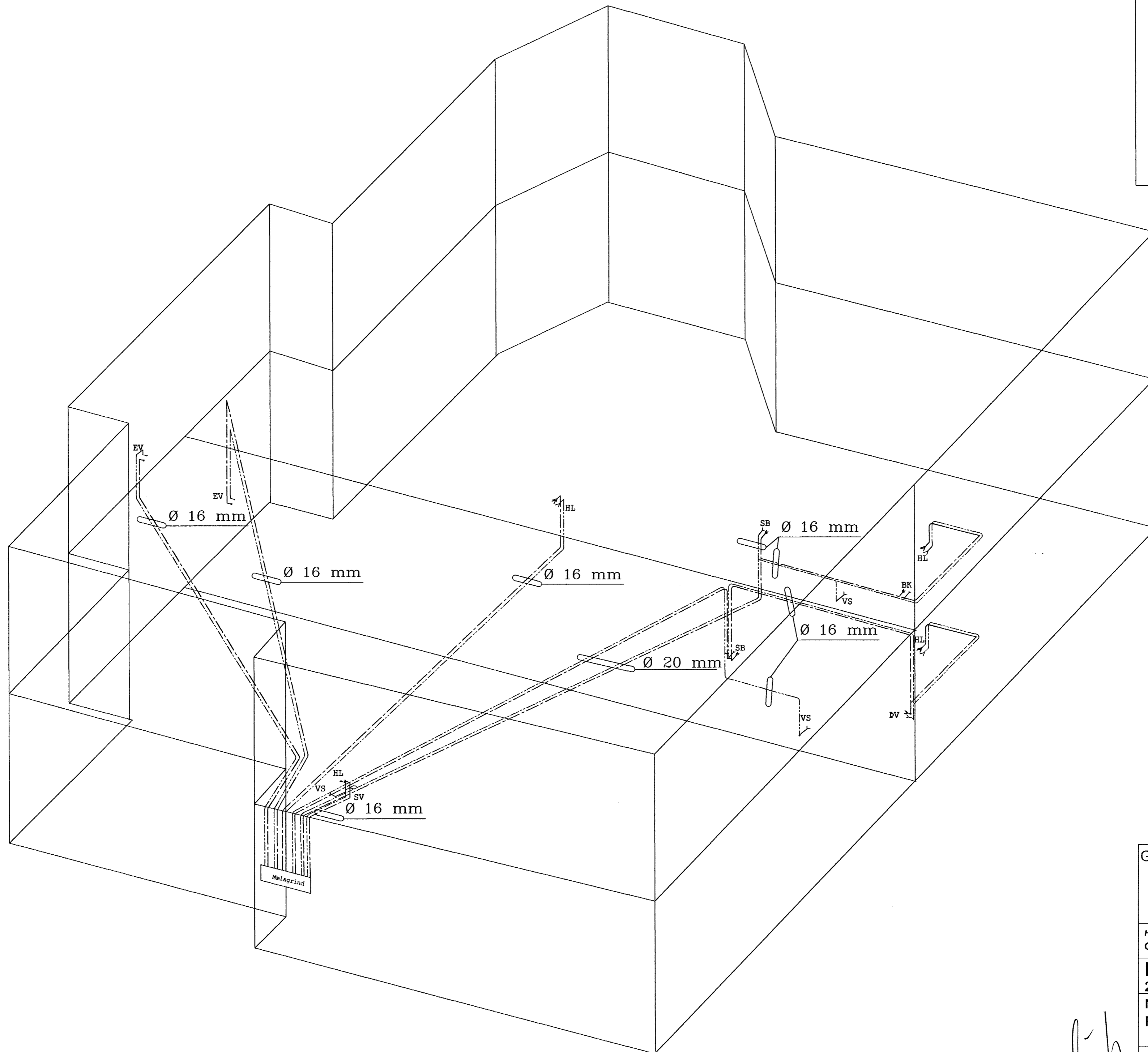
Rúmmynd neysluvatnslagnir
