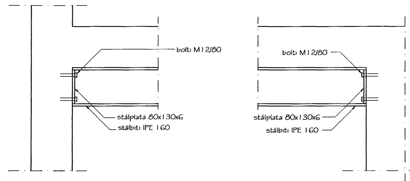
SÖGUN Á VEGG MILLI FORSTOFU OG ELDHÚSS - STYRKING Mkv. 1:10
