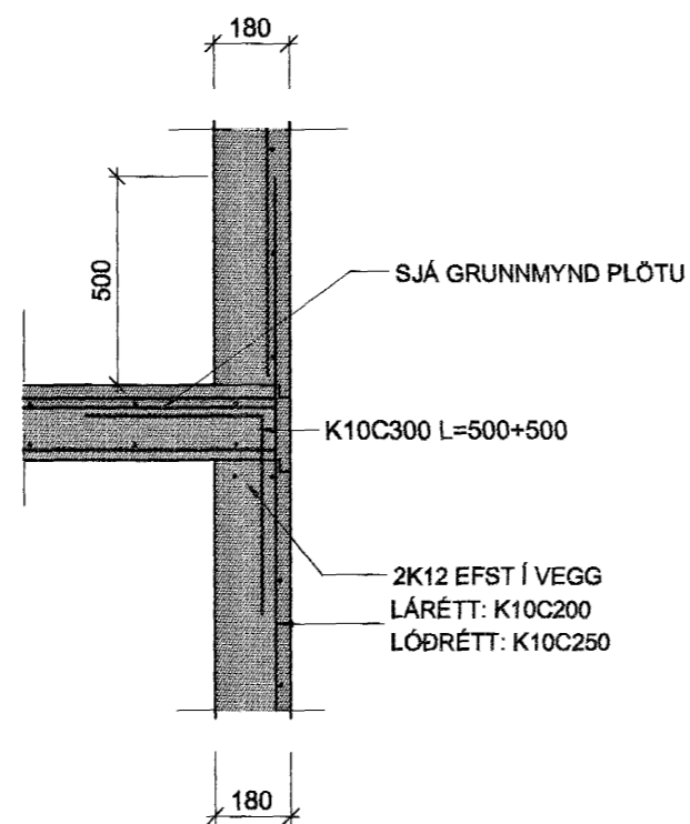
SNID D-D 1:20
