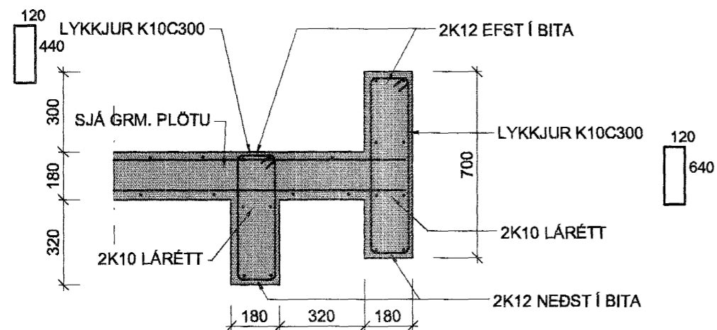
SNID A-A 1:20
