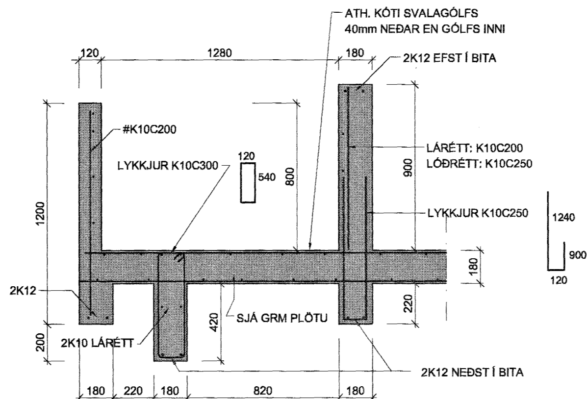
SNID B-B 1:20
