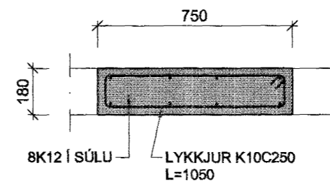
SÚLA S1 1:20
