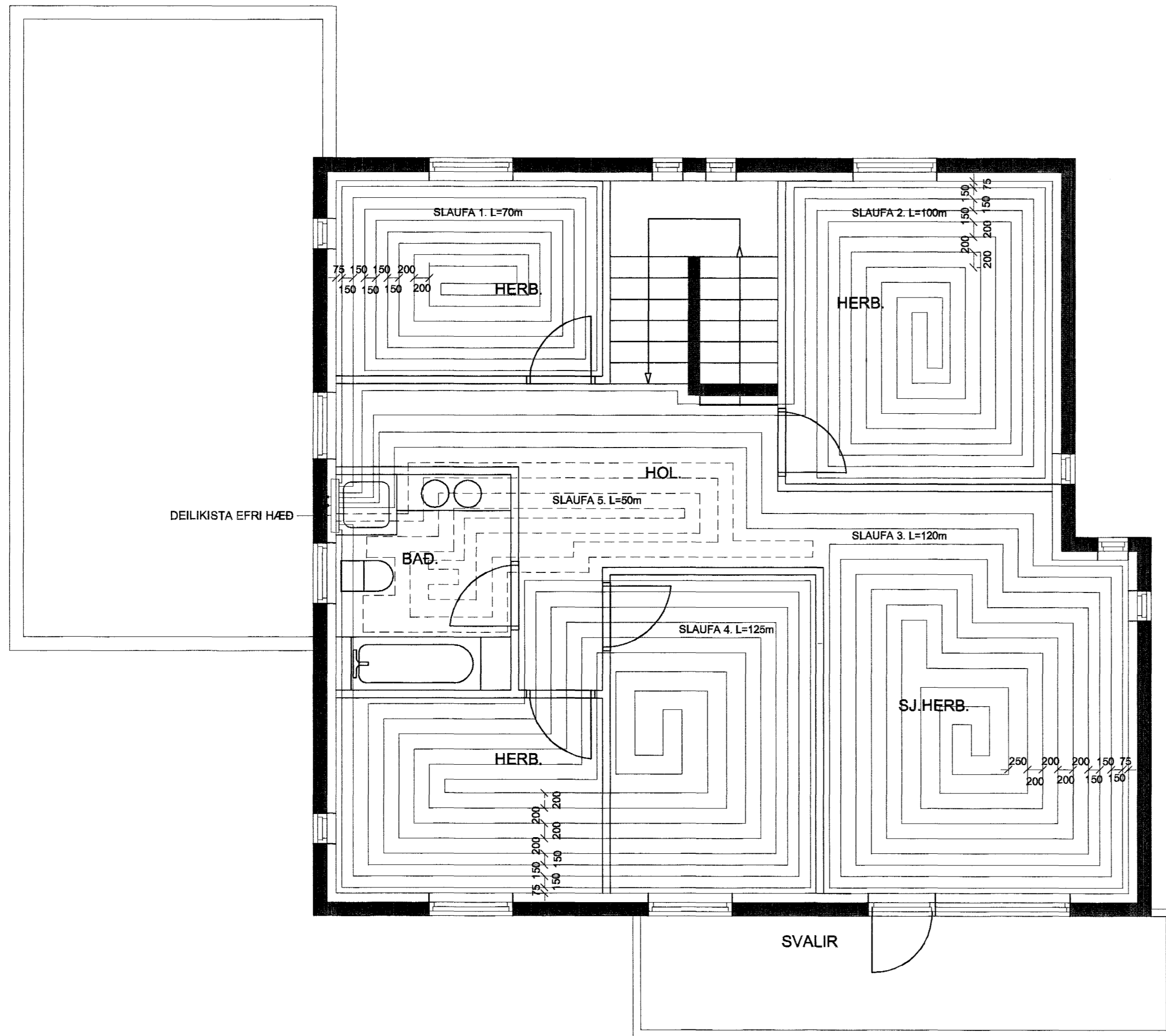
GRUNNMYND GÓLFHITALAGNA 2. HÆÐ, 1:50
