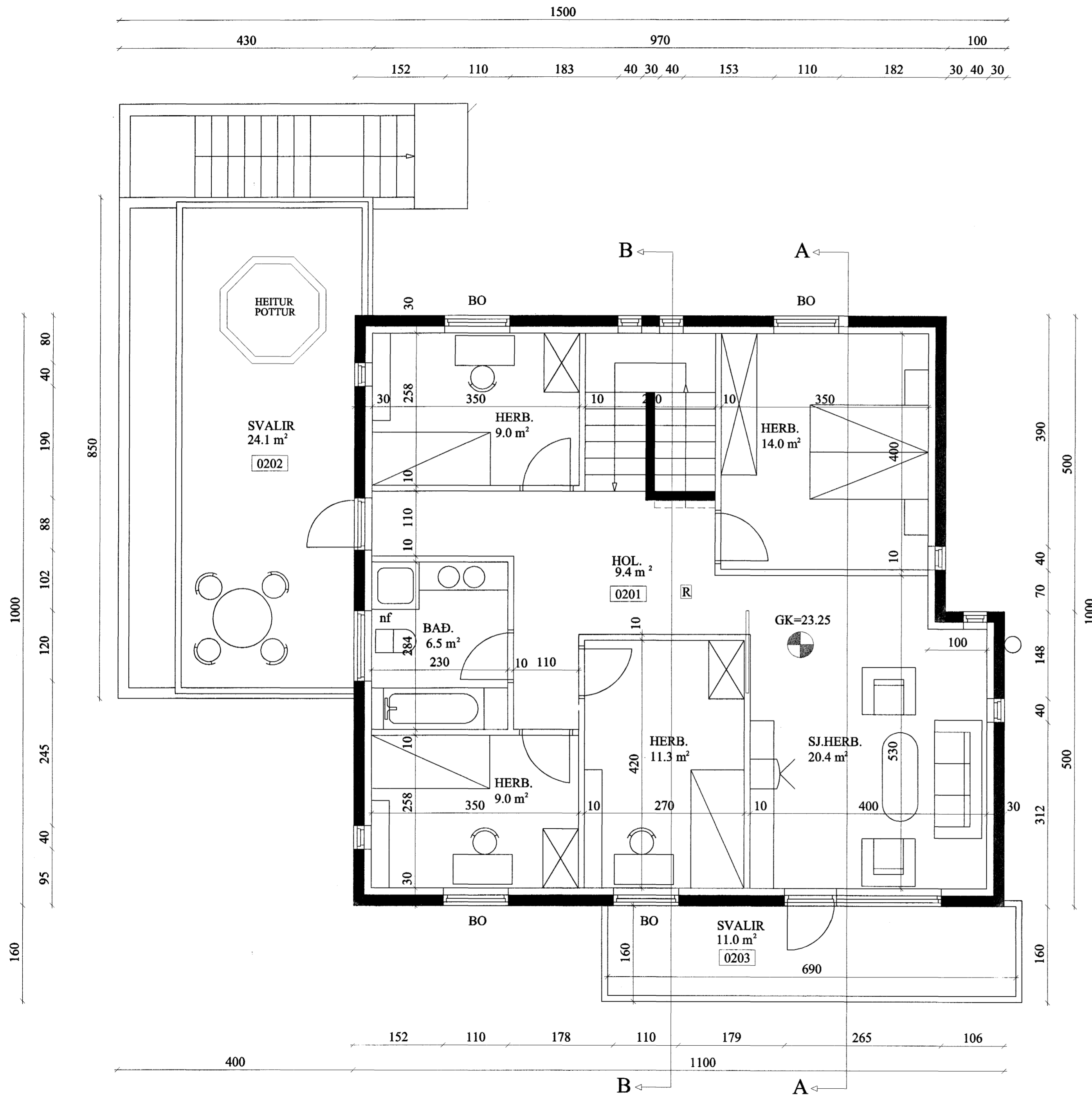
GRUNNMYND 2.HÆÐ.
