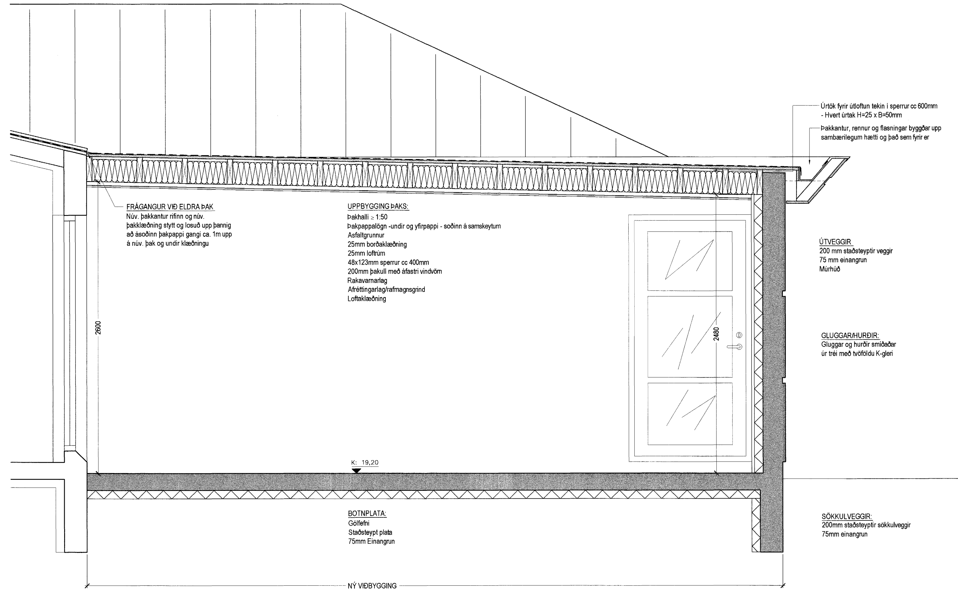
SNID A-A í mkv. 1:20
