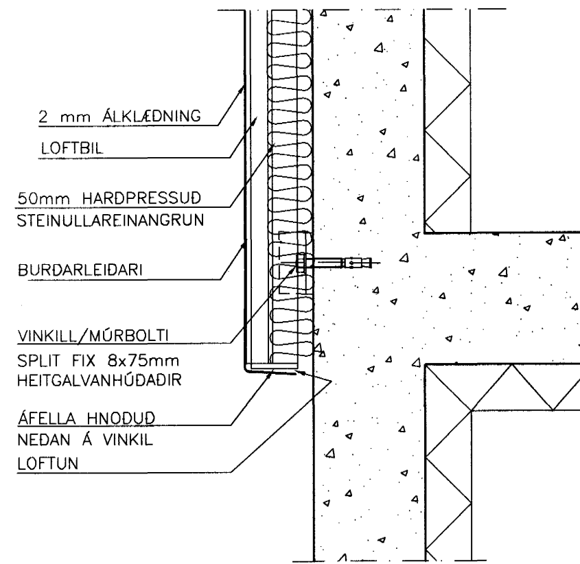
FRÁGANGUR VID JÖRD 1:5
