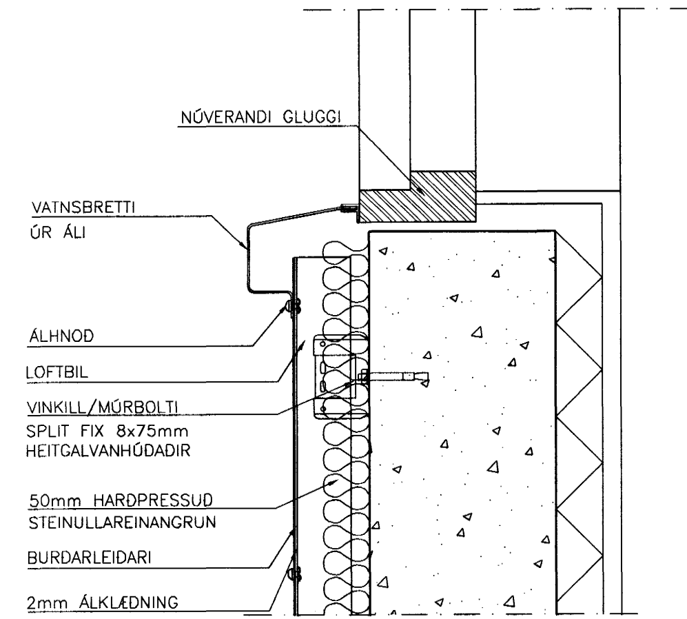
FRÁGANGUR UNDIR GLUGGUM 1:5
