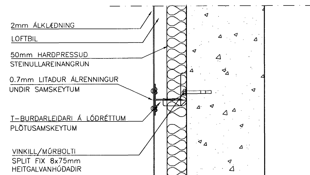
LÓDRÉTT PLÖTUSAMSKEYTI 1:5
