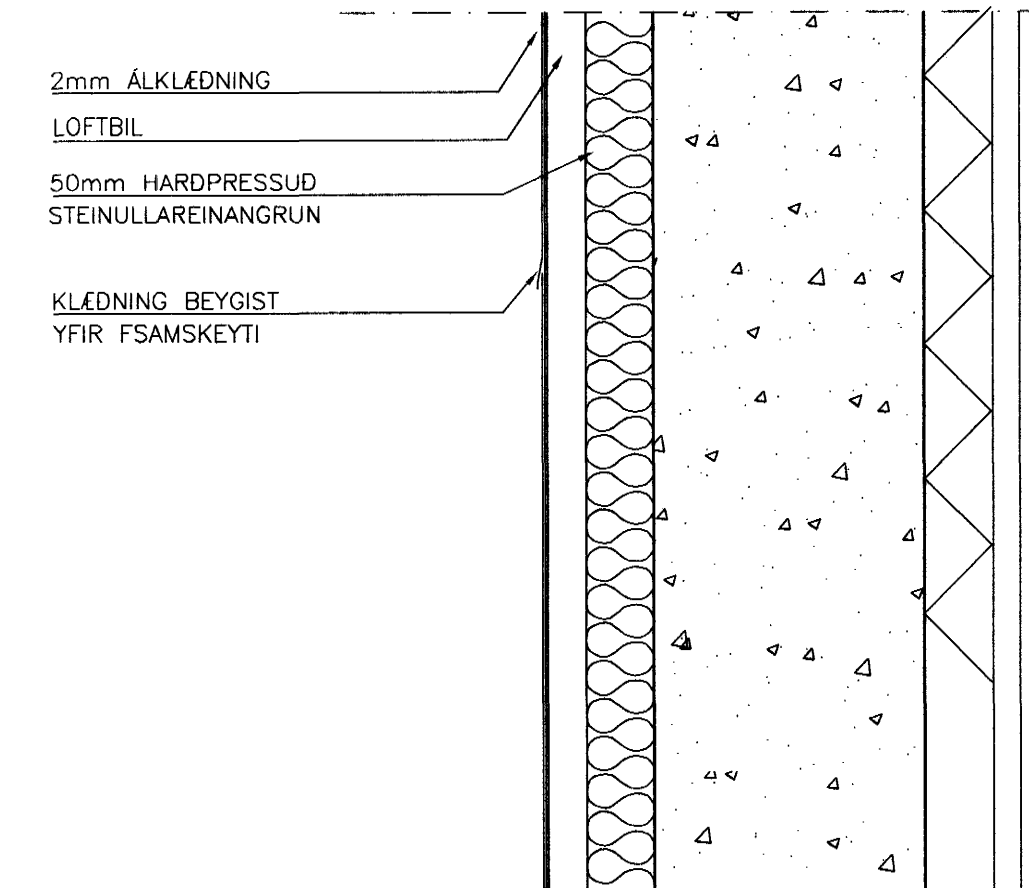
FRÁGANGUR Á LÁRÉTTUM PLÖTUSAMSKEYTUM 1:5
