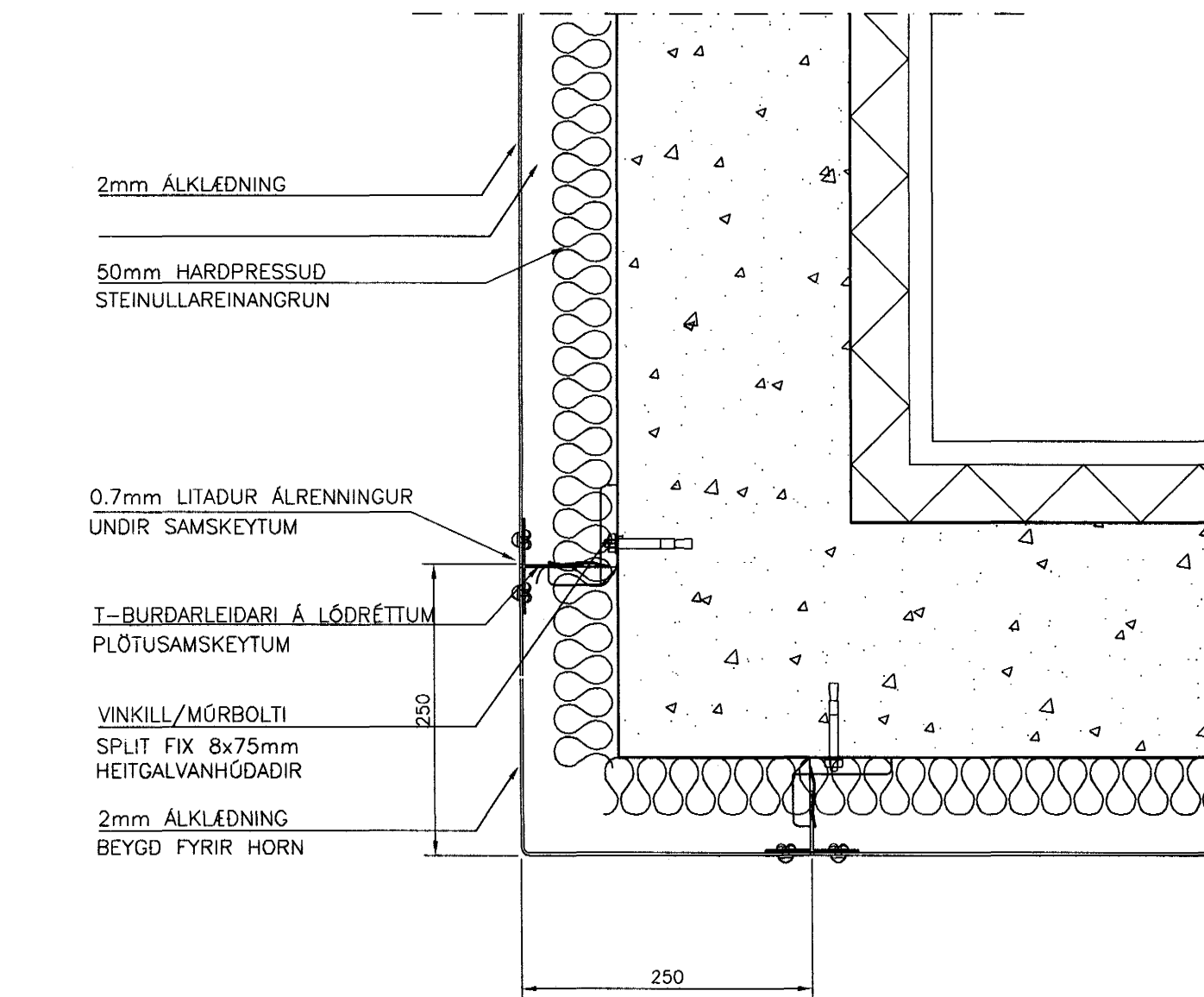
FRÁGANGUR Á ÓTHORNUM 1:5
