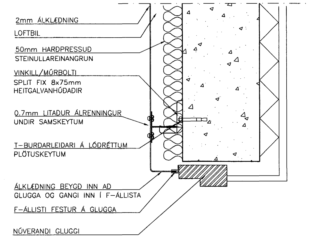
FRÁGANGUR VID GLUGGAHLIDAR 1:5
