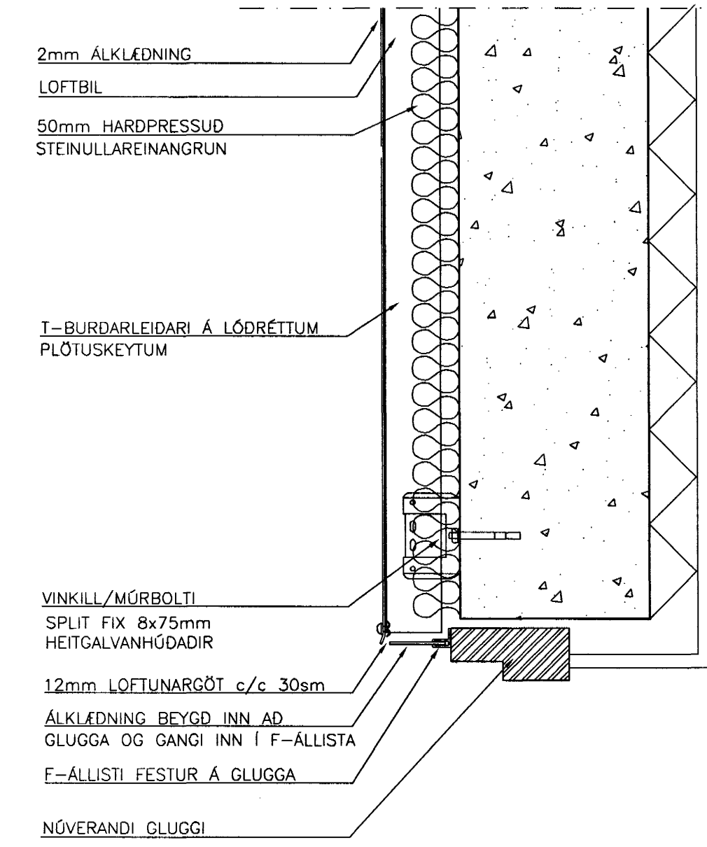
FRÁGANGUR OFAN VID GLUGGA 1:5
