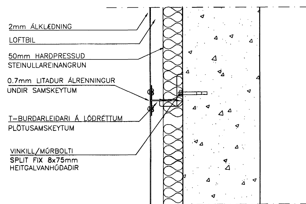
LÓDRÉTT PLÖTUSAMSKEYTI 1:5
