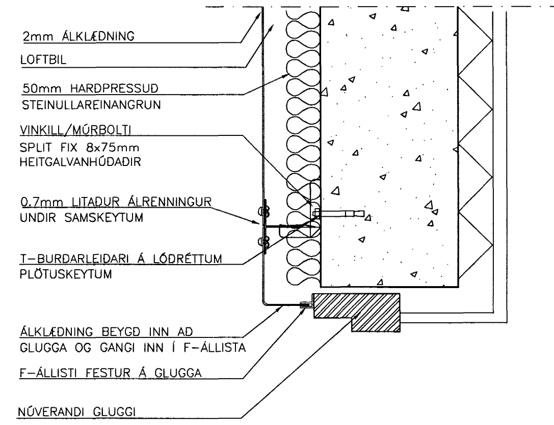
FRÁGANGUR VID GLUGGAHLIDAR 1:5
