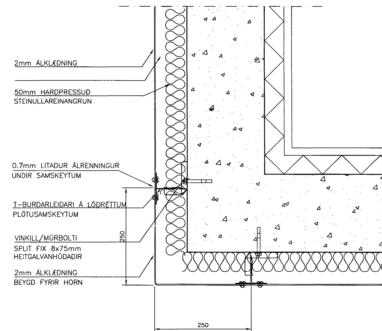
FRÁGANGUR Á ÚTHORNUM 1:5
