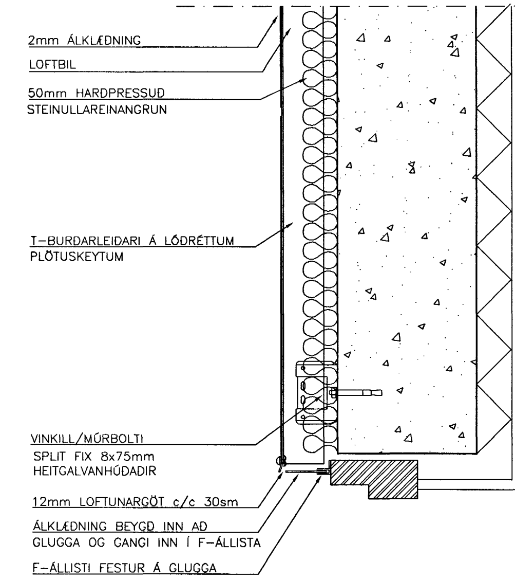
FRÁGANGUR OFAN VID GLUGGA 1:5
