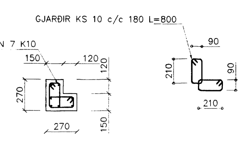
SÚLA S1 1:20
